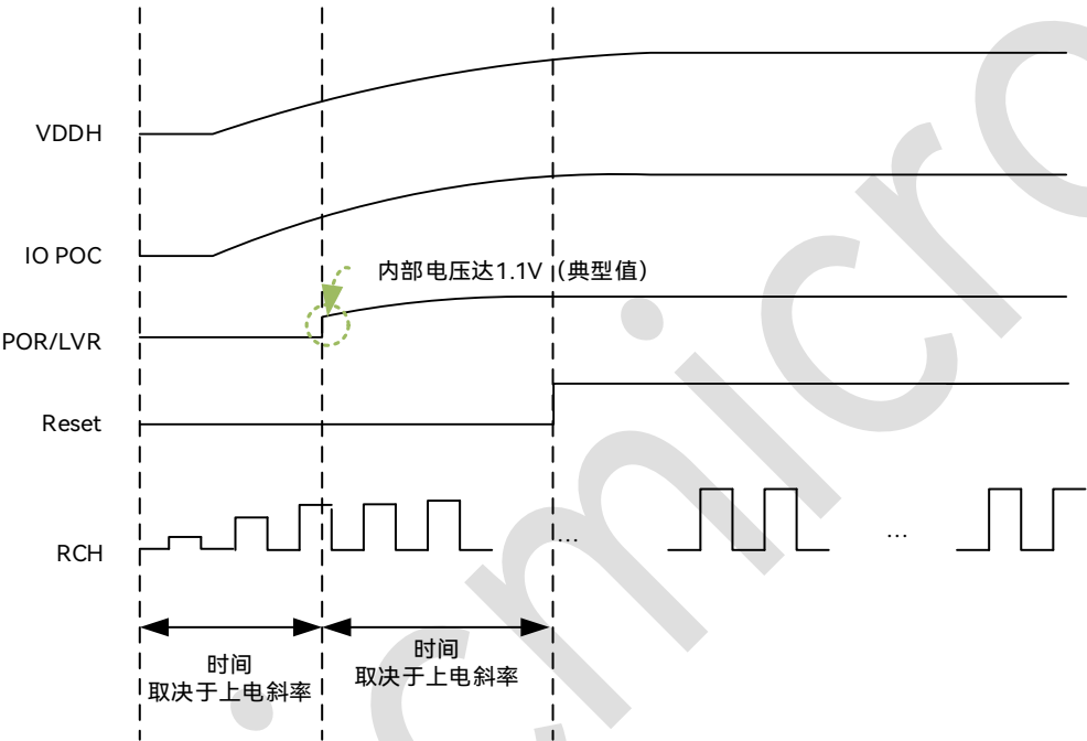
图 4-2：上电时序图
