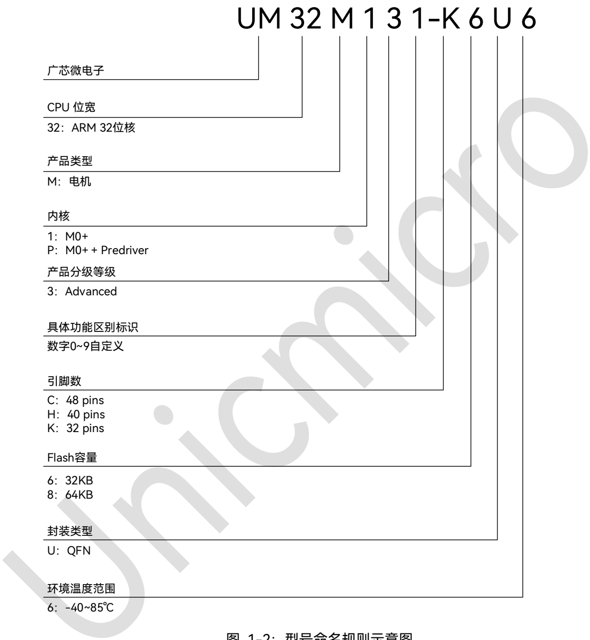
图 1-2：型号命名规则示意图
