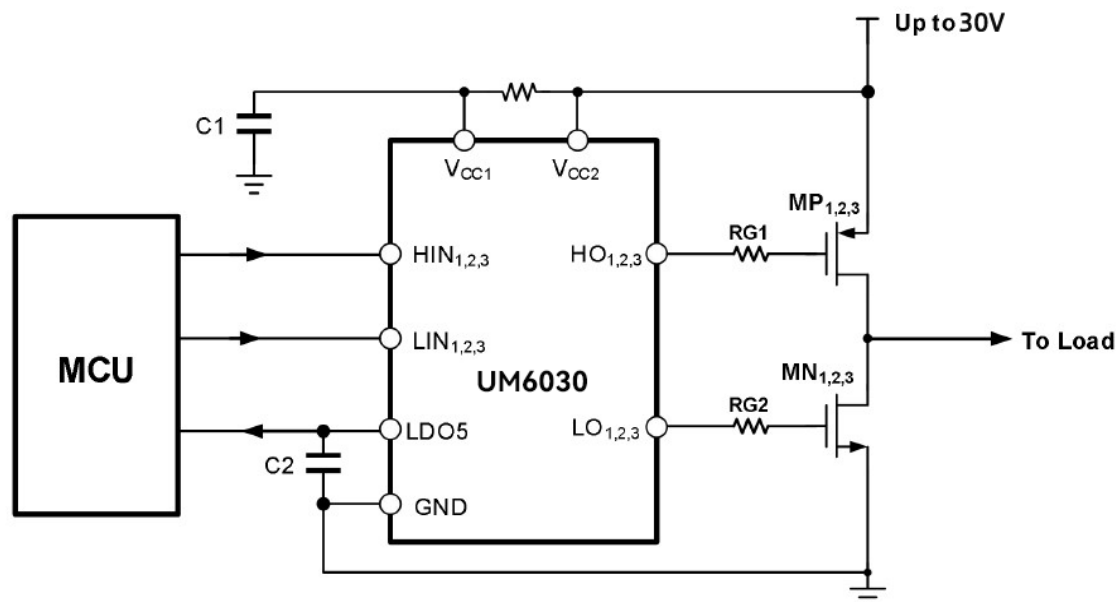
图 6-1: UM32MP32-H8U6 典型应用电路图
