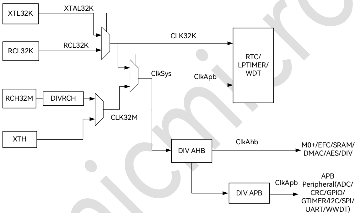
图 2-1：时钟架构图
