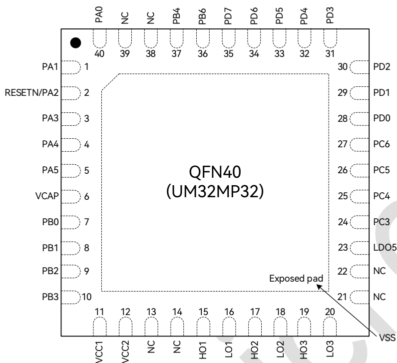
图 3-2: QFN40 引脚分布图
