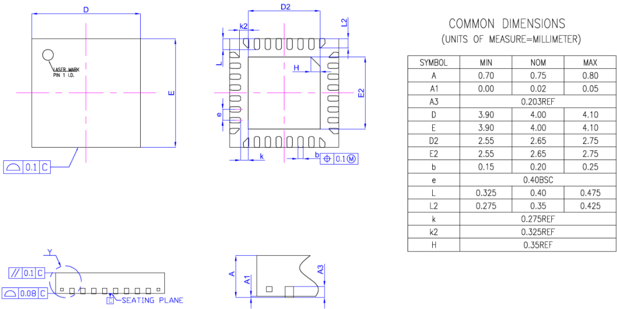
图 5-3: QFN32 封装尺寸图
