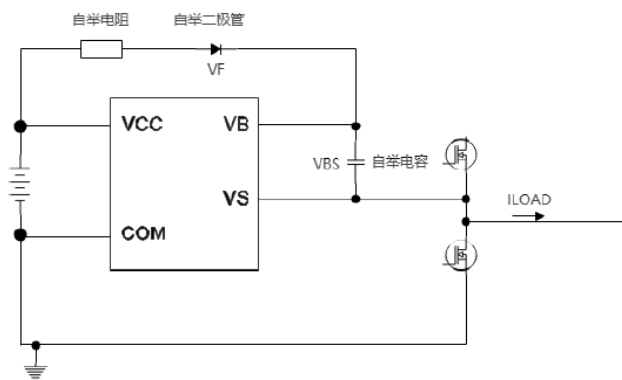
图 7-2: 自举电路基本结构
