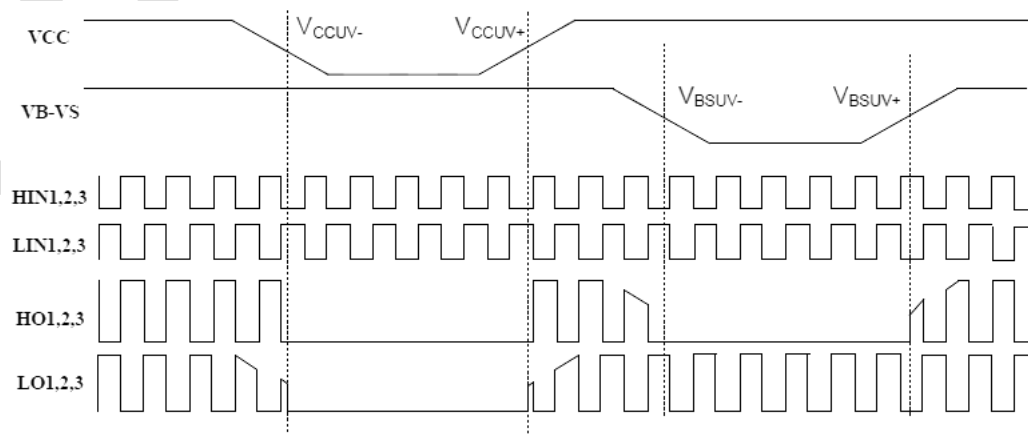
图 6-1: 欠压功能波形定义
