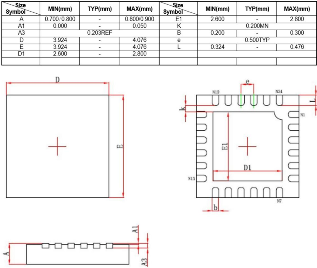
图 8-1：QFN24 封装尺寸图
