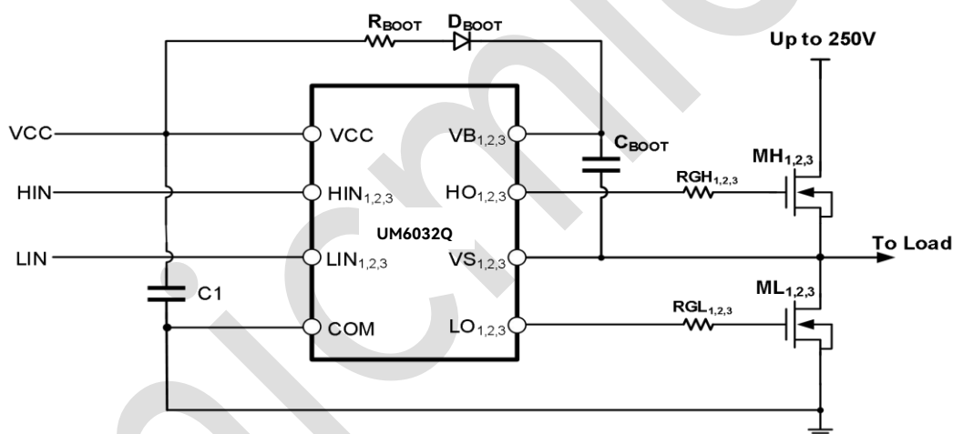
图 7-1：典型应用电路图
