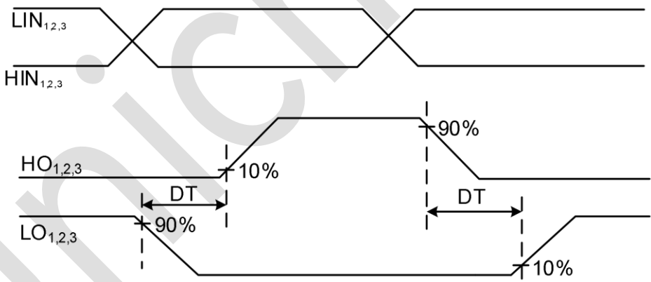
图 5-2: 死区时间波形定义
