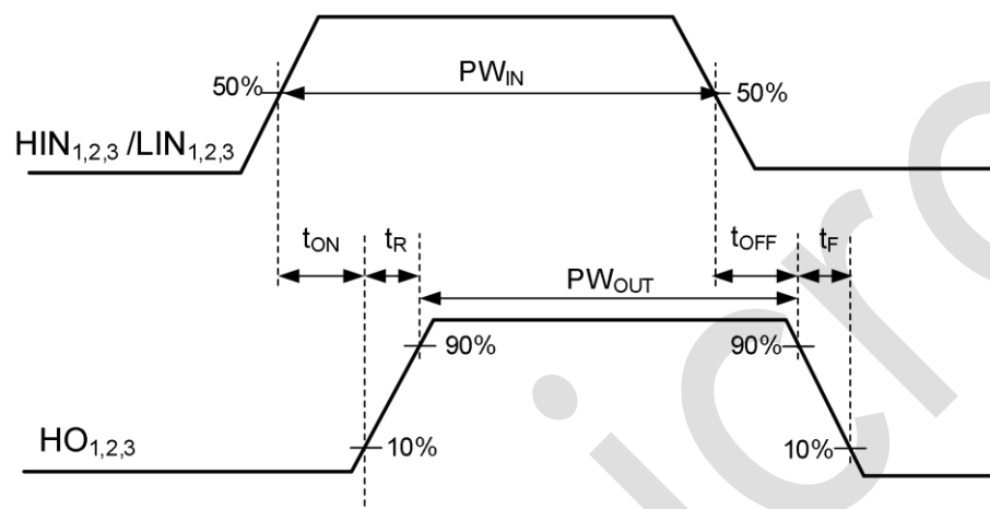
图 5-1: 传输延时波形定义
