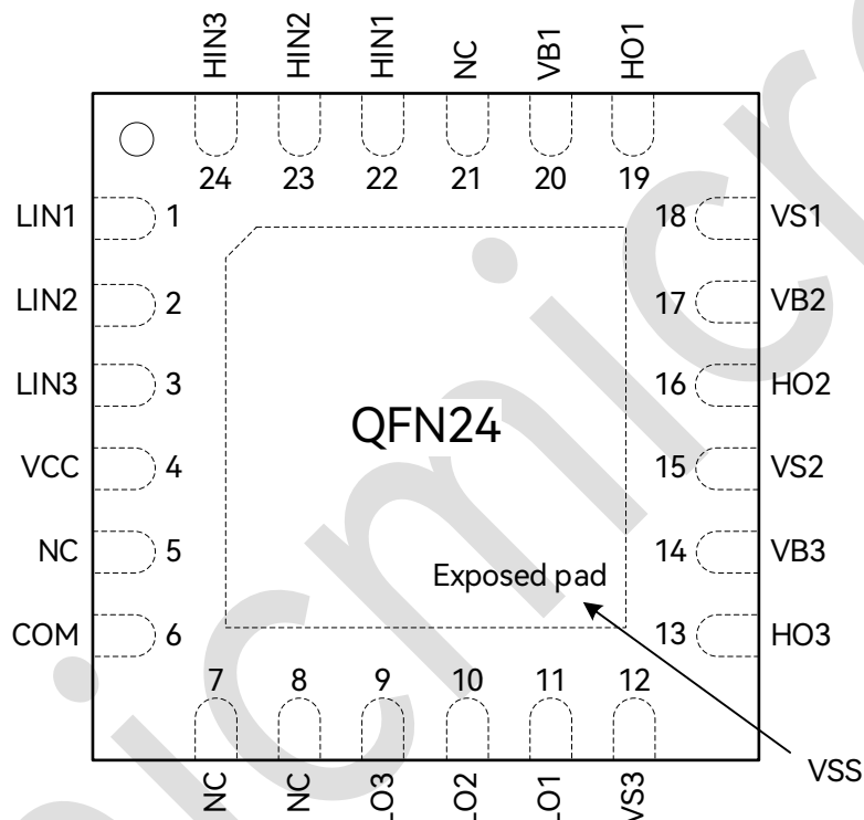
图 3-1：QFN24 封装引脚分布图
