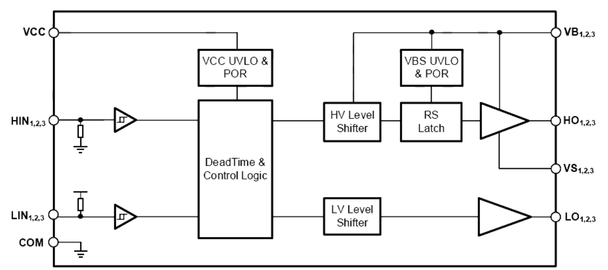
图 2-1：功能框图
