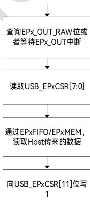
图 35-3: USB Endpoint Out 传输流程图
