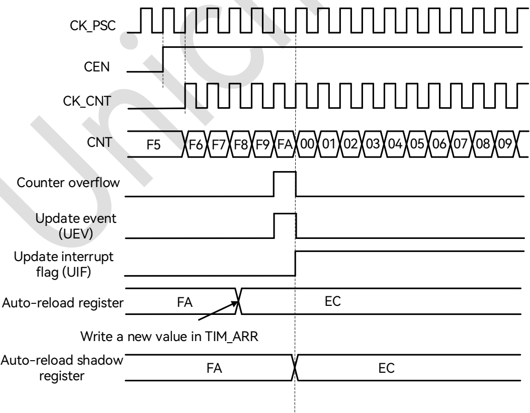
图 18-7: ARPE=1 (TIM_ARR 预装载) 时的更新事件图
