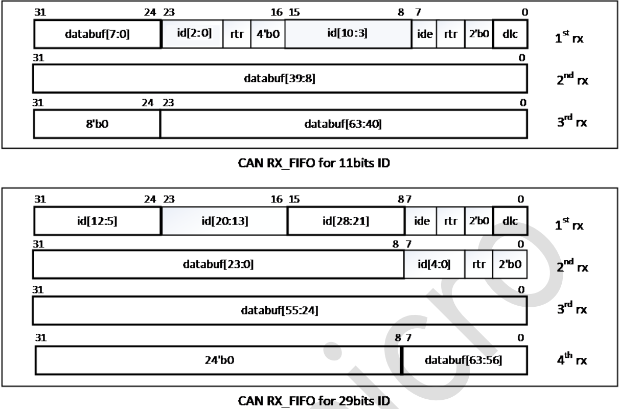
图 25-2: RXBUF 寄存器数据格式
