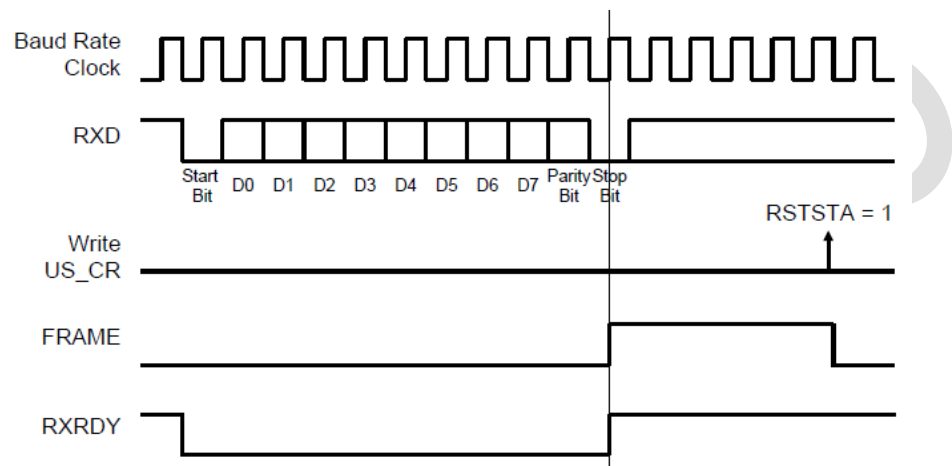
图 30-19：帧错误状态时序图
