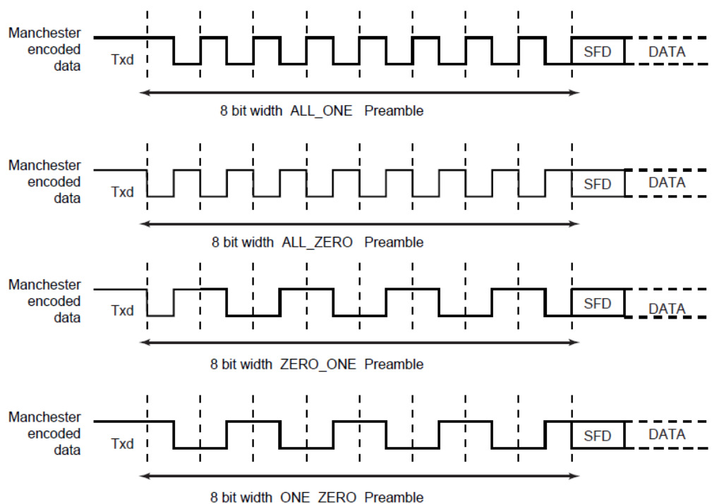
图 30-4：前同步信号模式
