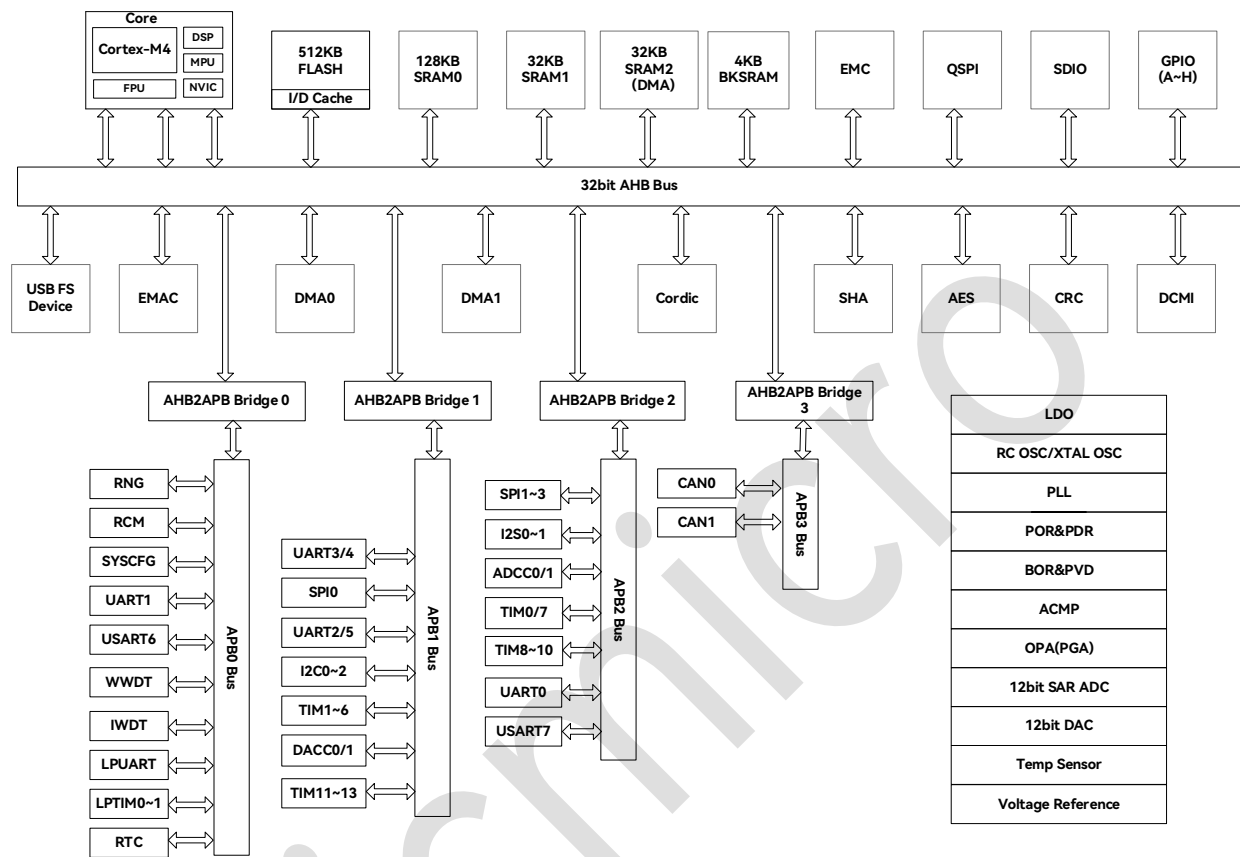
图 3-1: 总线架构图
