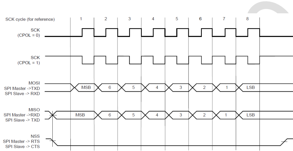
图 30-27: SPI 传输格式 (CPHA=1, 每次传输 8 位)
