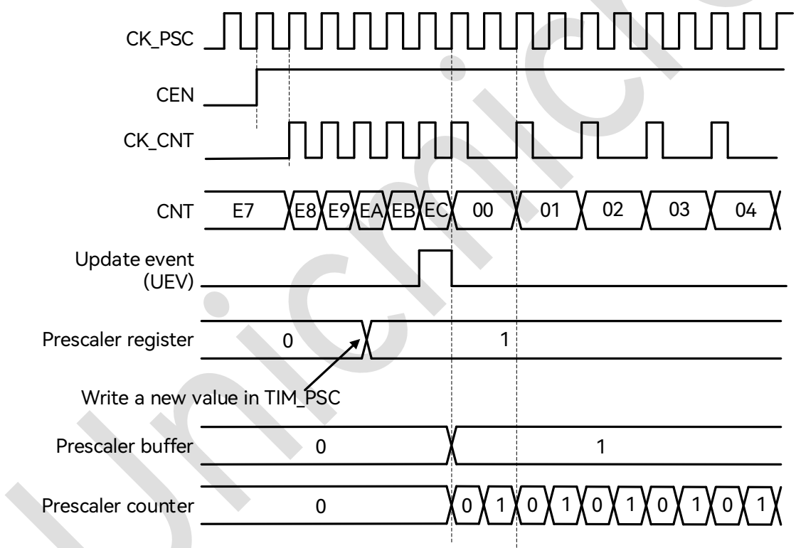
图 20-1: 预分频从 1 变为 2 的波形
