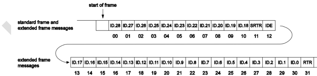
图 25-7：仲裁丢失位中断图
