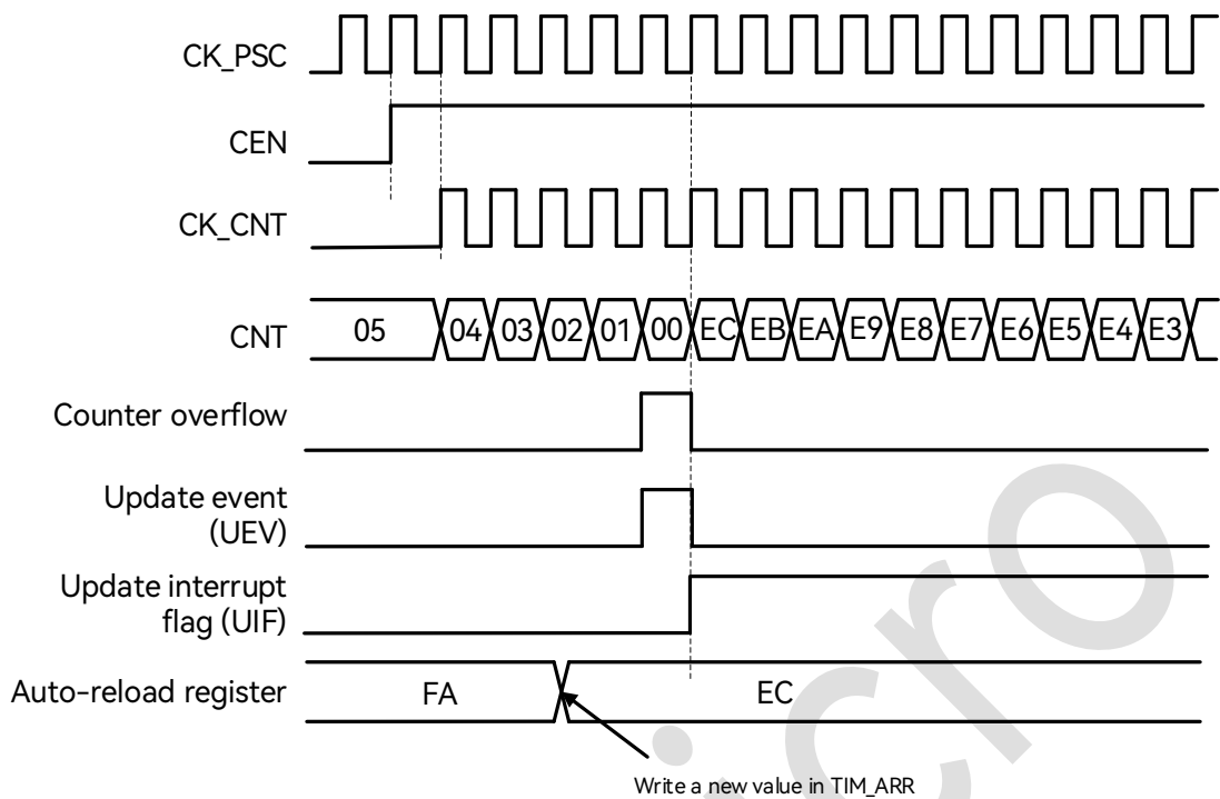
图 19-10: 向下计数，内部时钟 2 分频
