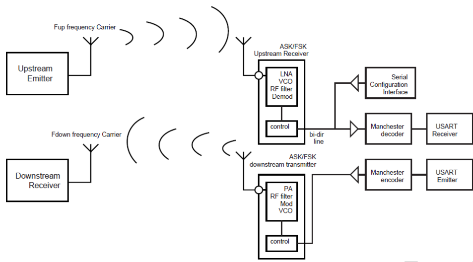
图 30-12：曼彻斯特编码字符射频传输图
