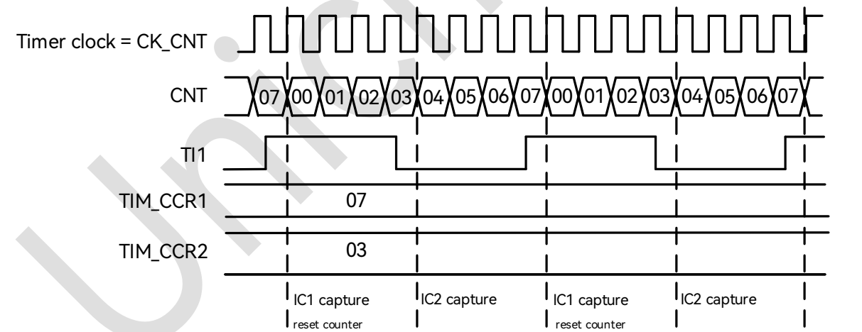
图 19-26：PWM 输入捕获模式时序
