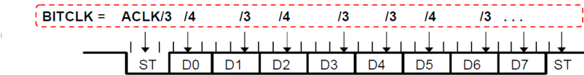
图 29-3：LPUART 接收时序图
