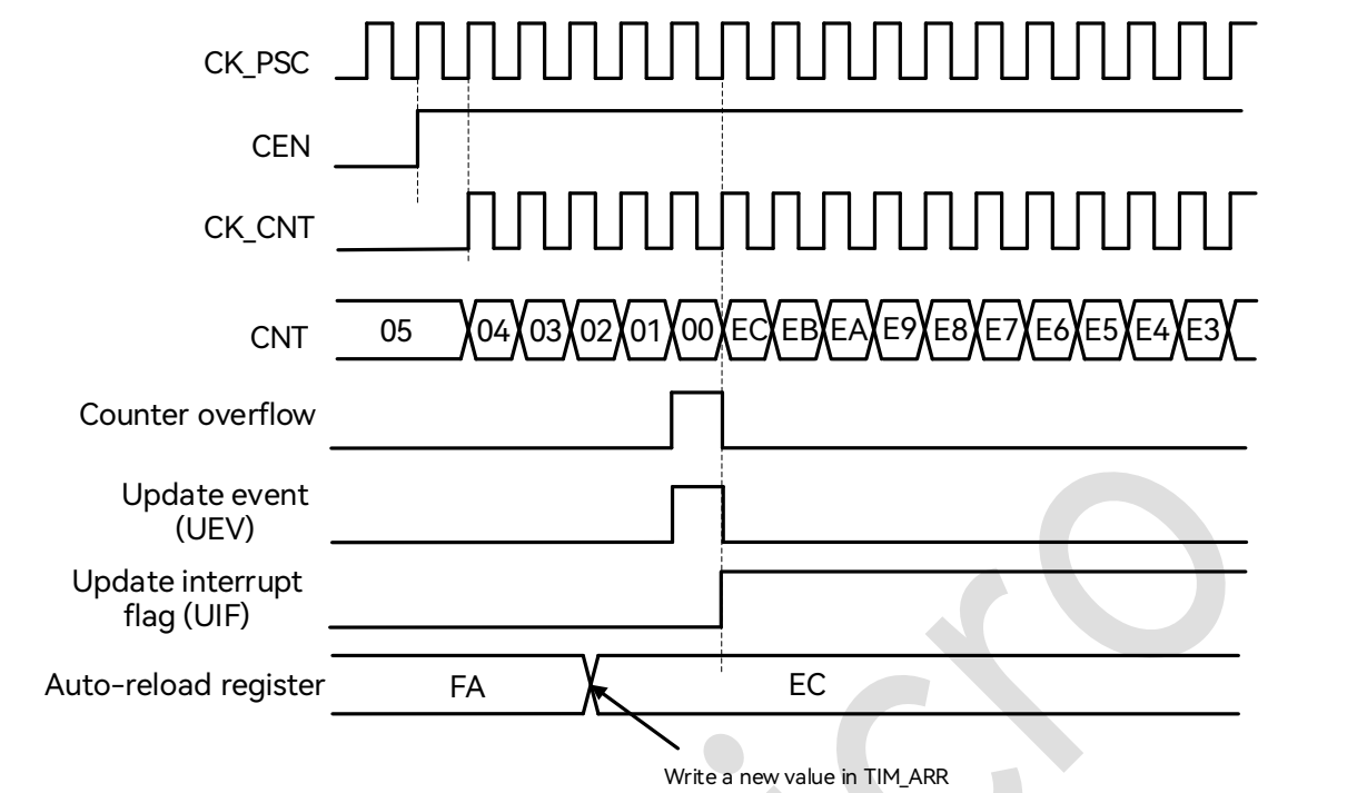
图 18-11: 向下计数，不使用重复计数时的更新事件图
