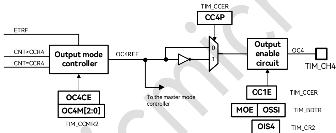
图 19-25: 捕获/比较通道的输出部分 (通道 4)
