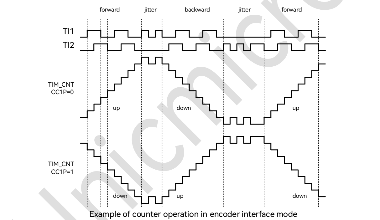
图 19-32：编码器模式下的计数器操作实例
