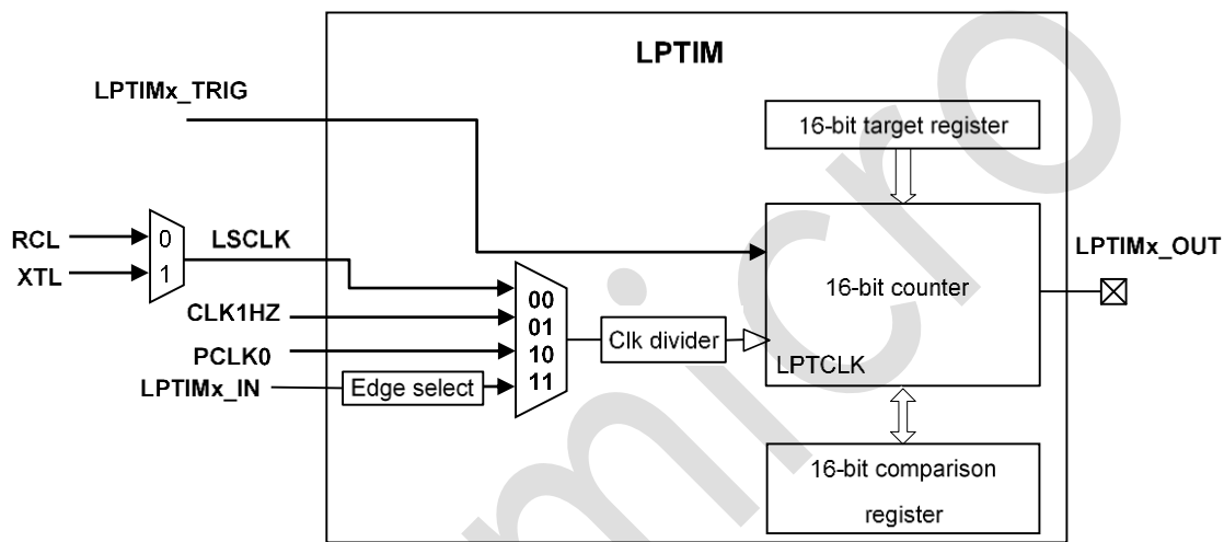
图 21-1：系统框图
