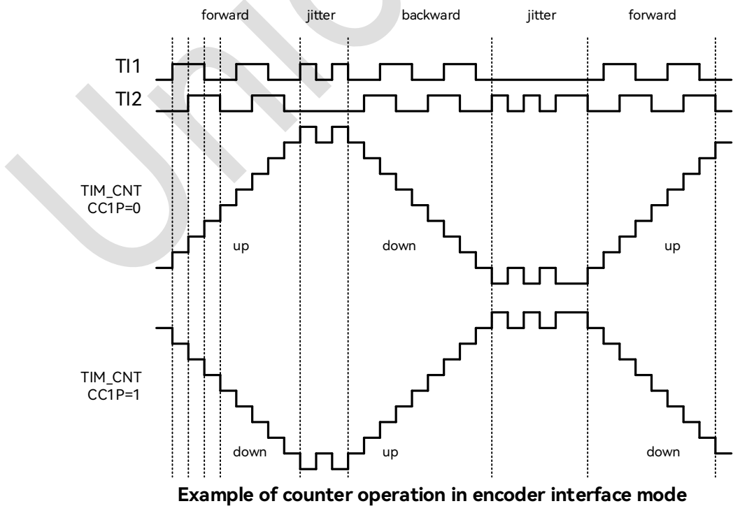
图 18-38: 编码器模式下的计数器操作实例图
