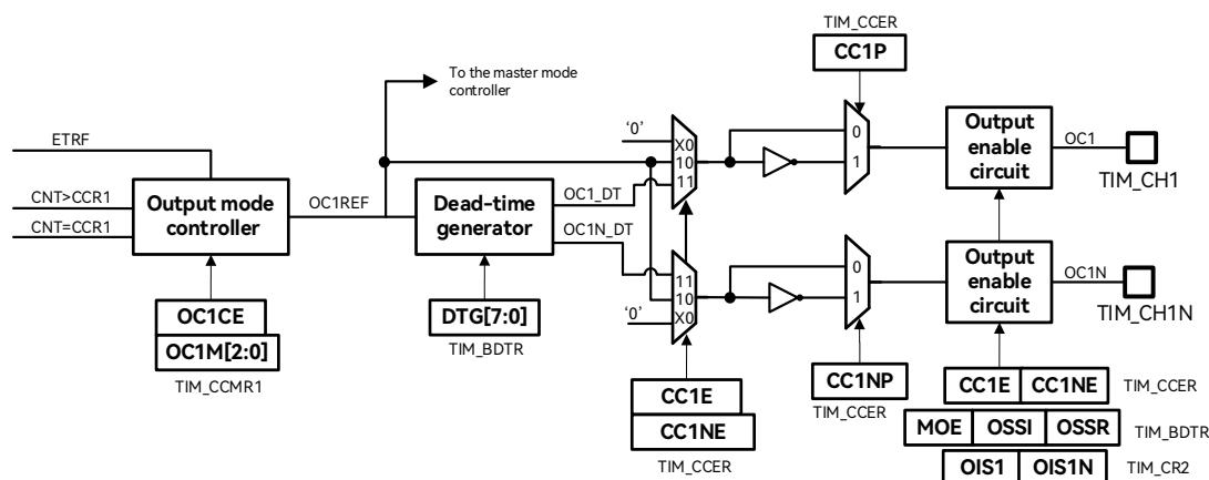
图 19-24: 捕获/比较通道的输出部分 (通道 1 至 3)
