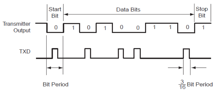
图 30-25: IrDA 调制
