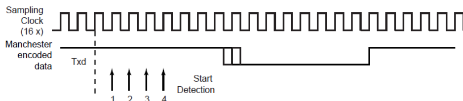
图 30-9: 异步起始位检测
