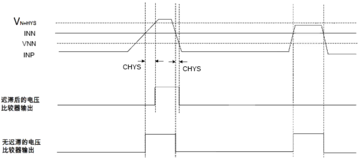
图 38-3：带迟滞功能的电压比较功能图
