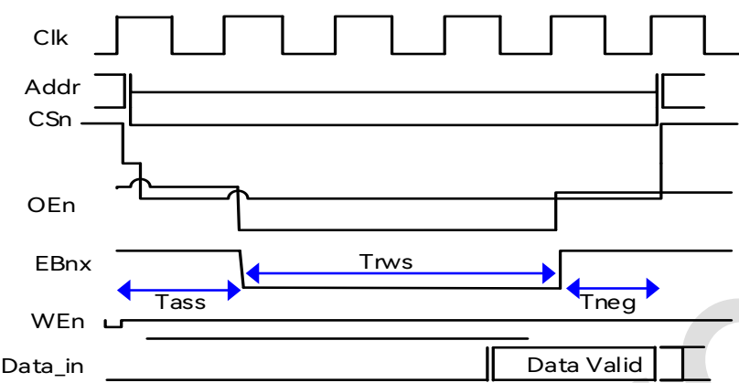
图 13-2: 片外存储控制器读操作时序图
