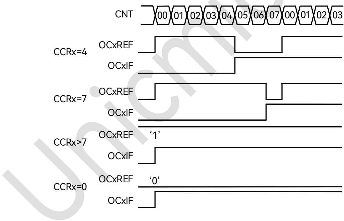
图 18-29：边沿对齐的 PWM 波形（ARR=7）图
