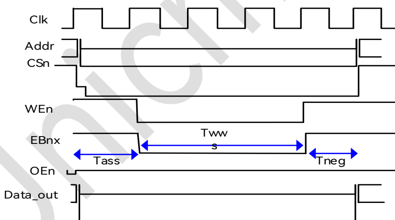
图 13-1: 片外存储控制器写操作时序图
