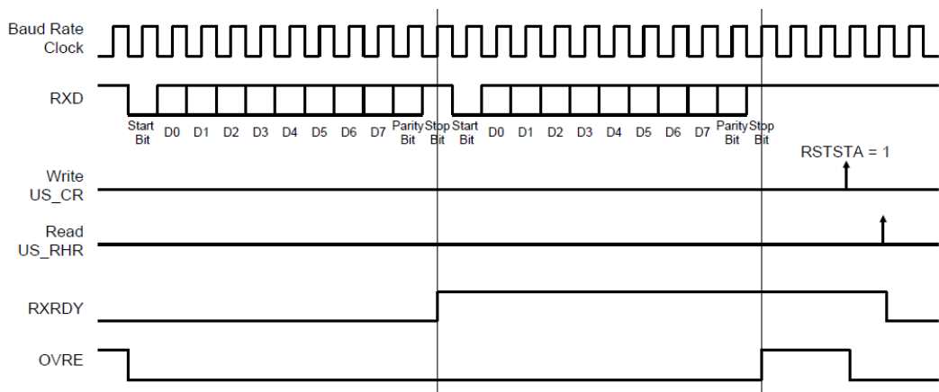
图 30-16：接收器状态
