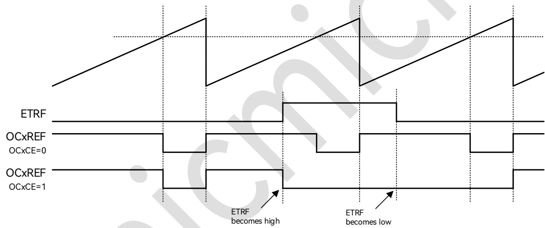
图 19-31: ETR 信号清除 TIM 的 OCxREF
