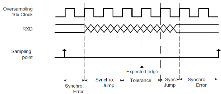
图 30-6：位同步图
