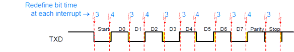
图 29-4：LPUART 发送时序图
