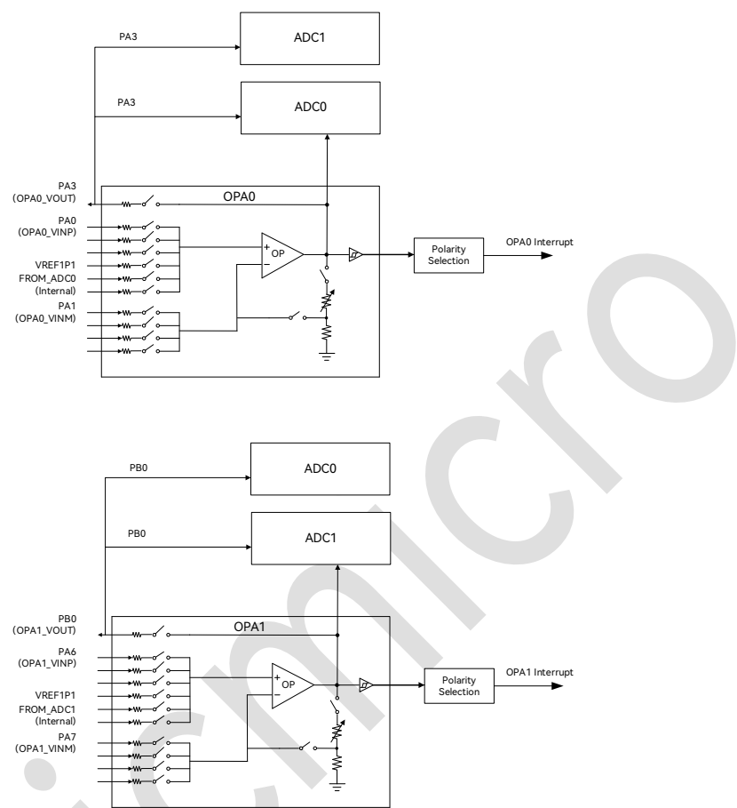
图 39-1: OPA 系统框图
