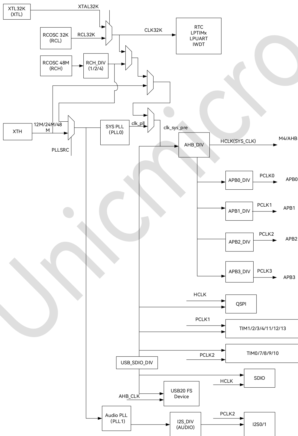
图 6-1: 时钟单元
