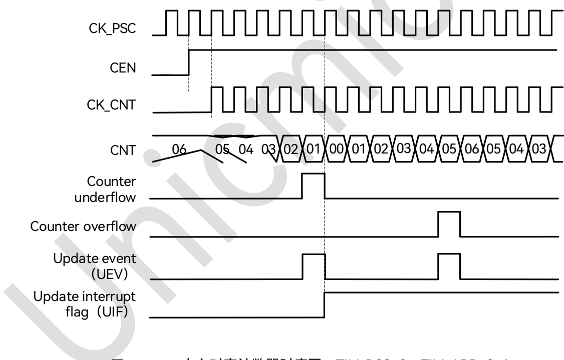
图 19-12: 中心对齐计数器时序图, TIM_PCS=0, TIM_ARR=0x6
