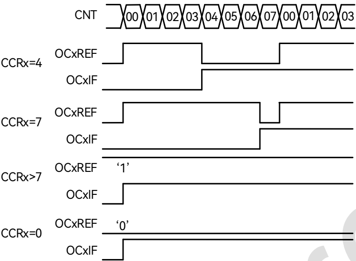
图 19-28: 边沿对齐的 PWM 波形 (ARR=7)
