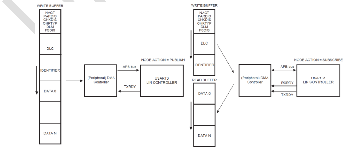
图 30-41：使用 DMA/PDC 的主节点 (PDCM=1)
