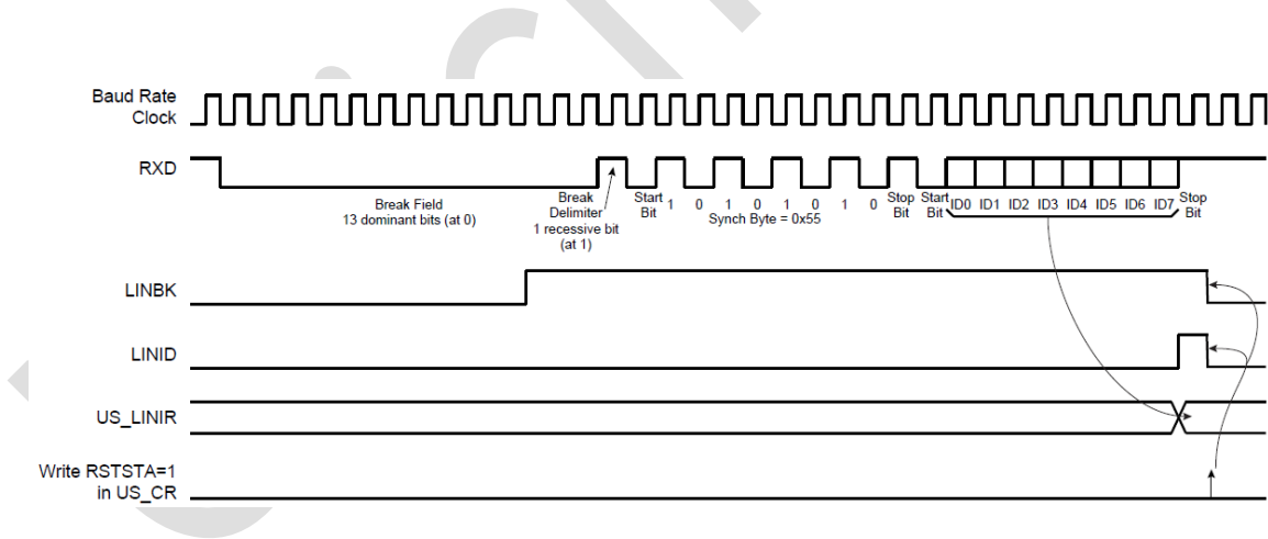
图 30-30：报文接收
