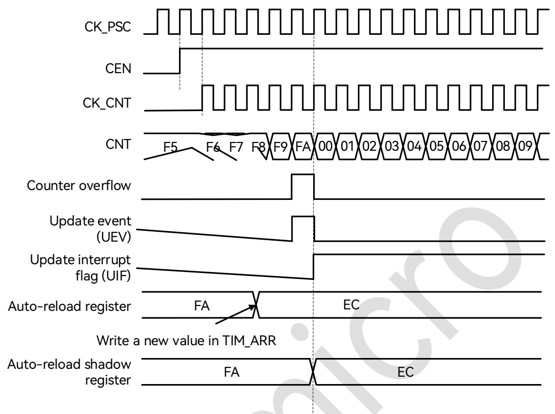
图 20-6: ARPE=1 (TIM_ARR 预装载) 时的更新事件
