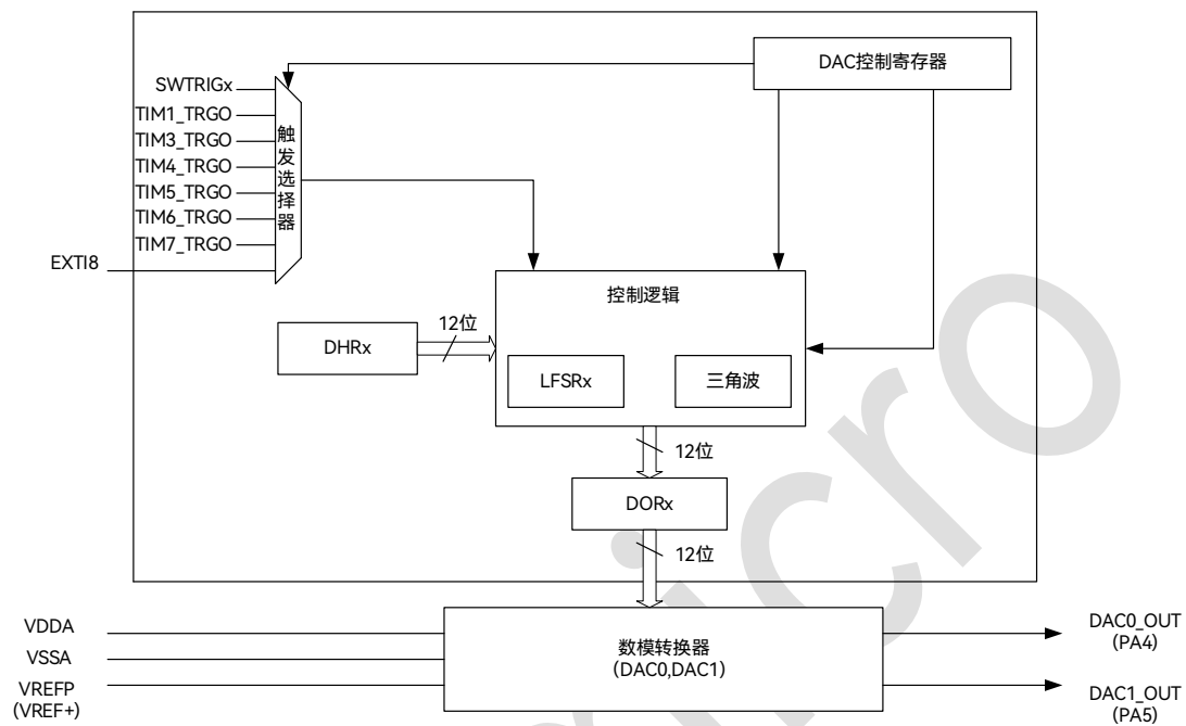
图 37-1: DAC 系统框图
