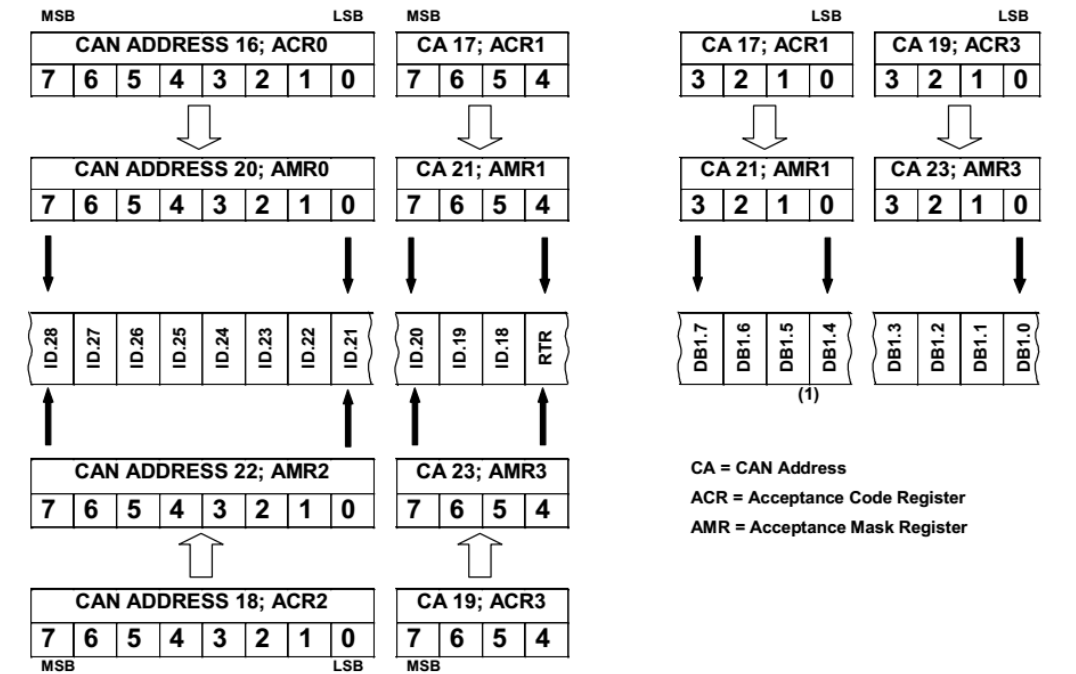
图 25-5：双过滤器标准帧对应位格式
