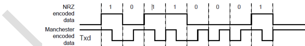
图 30-3: NRZ 码转为曼彻斯特码
