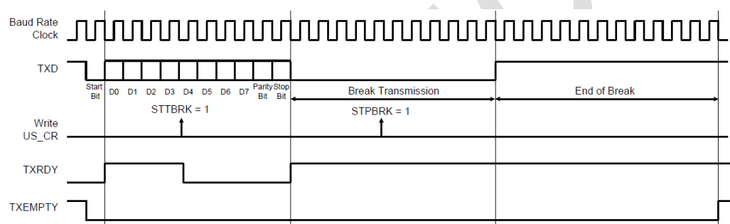
图 30-20：中断的传输
