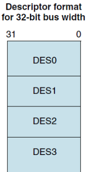
图 33-3: DES0 ~ DES3 结构图
