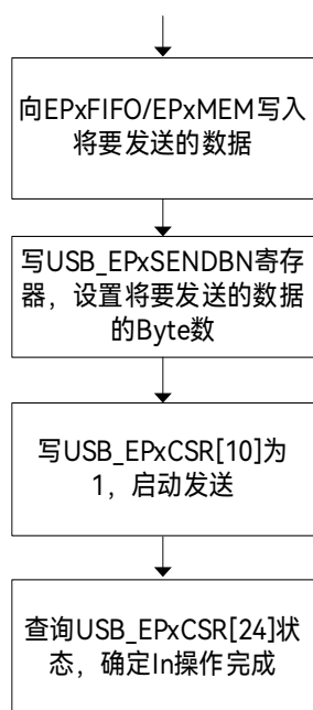
图 35-2: USB Endpoint In 传输流程图
