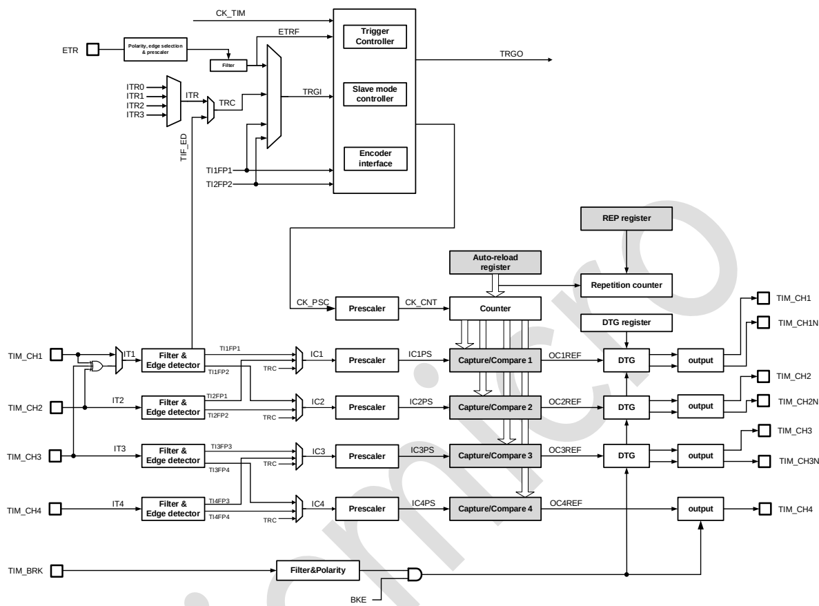
图 18-1: TIM0&TIM7 系统框图
