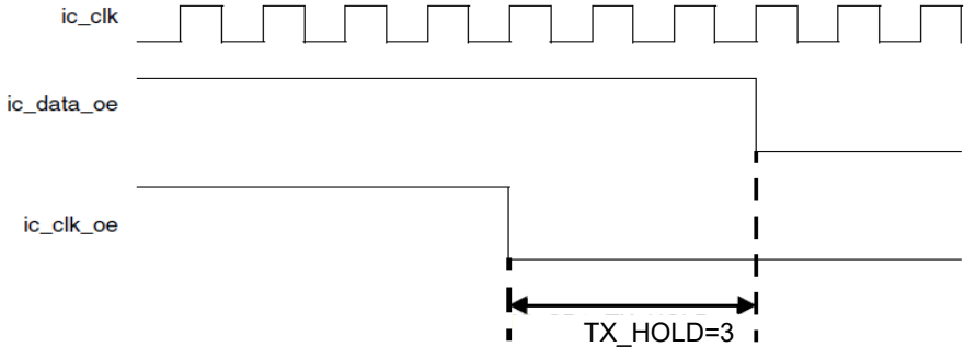
图 26-3: I2C 主机模式 TX_HOLD = 3 时序图
