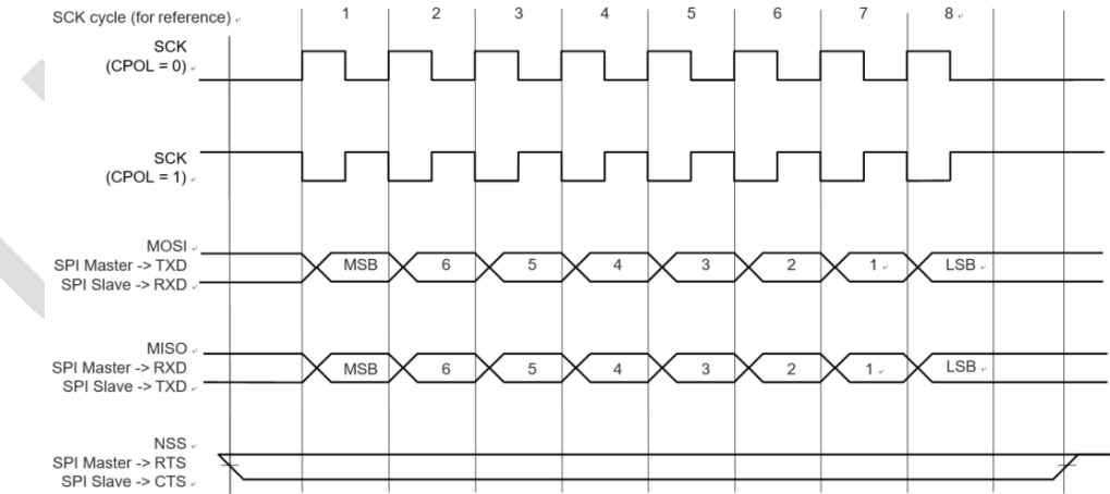
图 30-28: SPI 传输格式 (CPHA=0, 每次传输 8 位)
