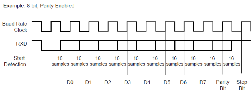
图 30-8：字符接收
