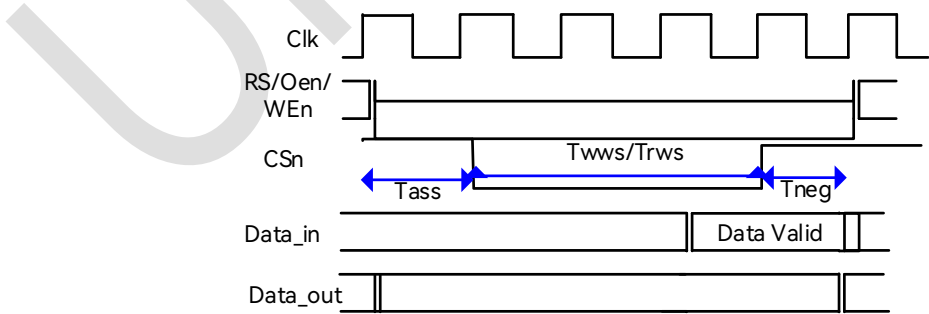
图 13-3: I8080 TFT-LCD 时序接口
