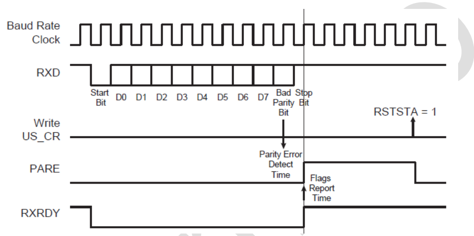
图 30-17：检验错误时序图
