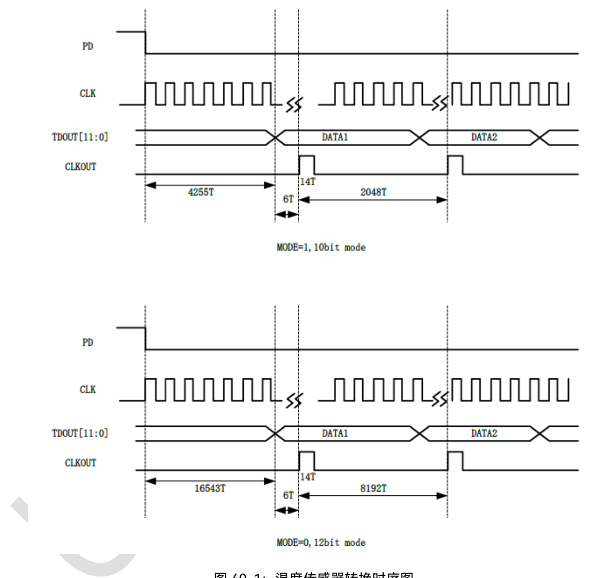
图 40-1：温度传感器转换时序图
