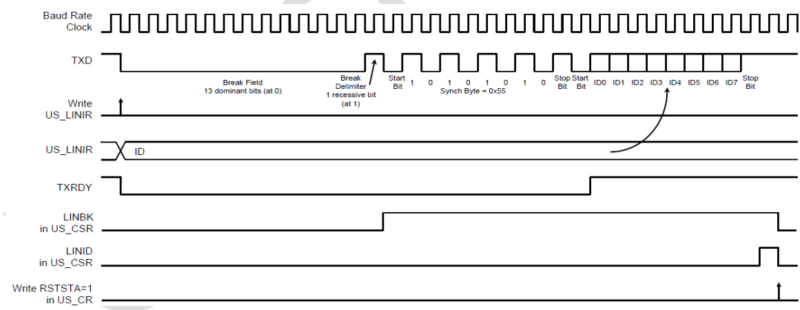
图 30-29：报文传输
