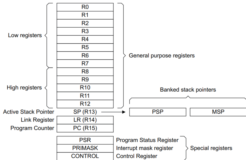
图 4-2: Cortex-M0+的寄存器组
