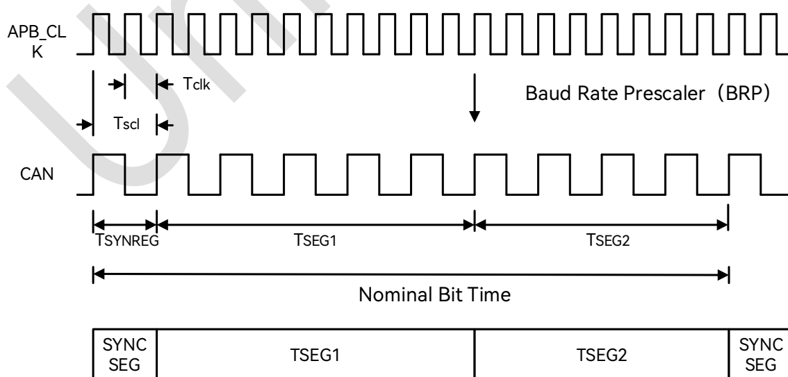
图 14-1: CAN 的位周期结构图
