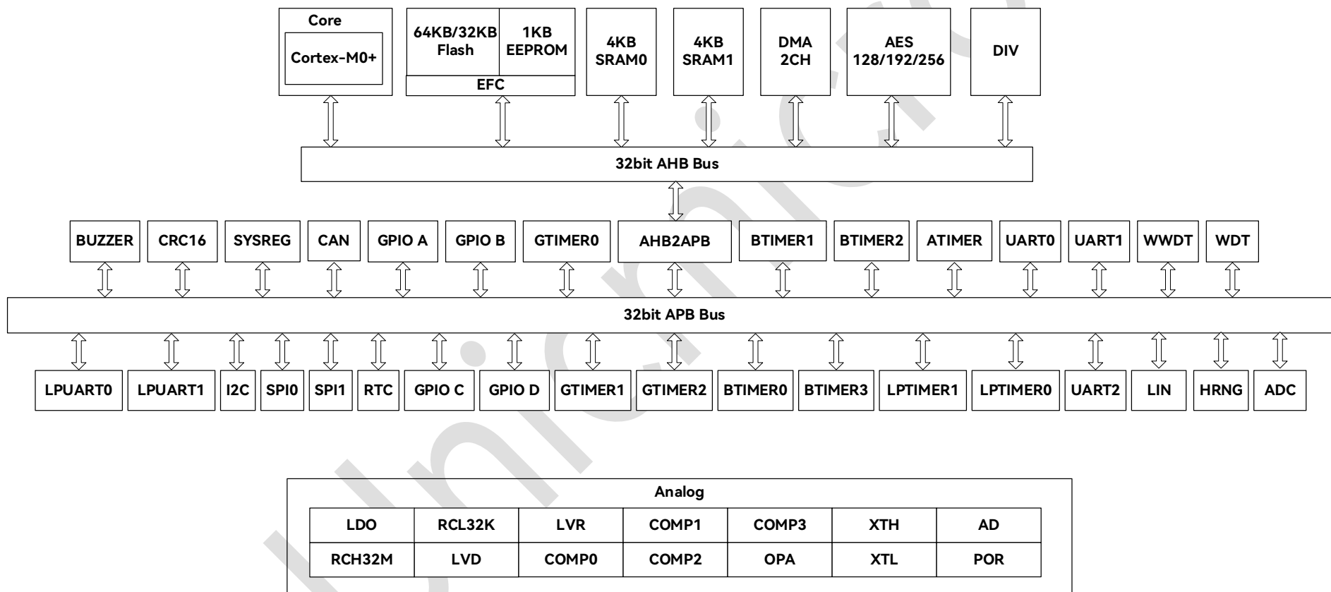
图 3-1: 总线架构图
