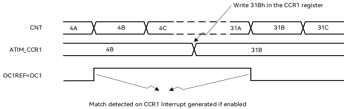
图 16-6: 输出比较模式, 翻转 OC1
