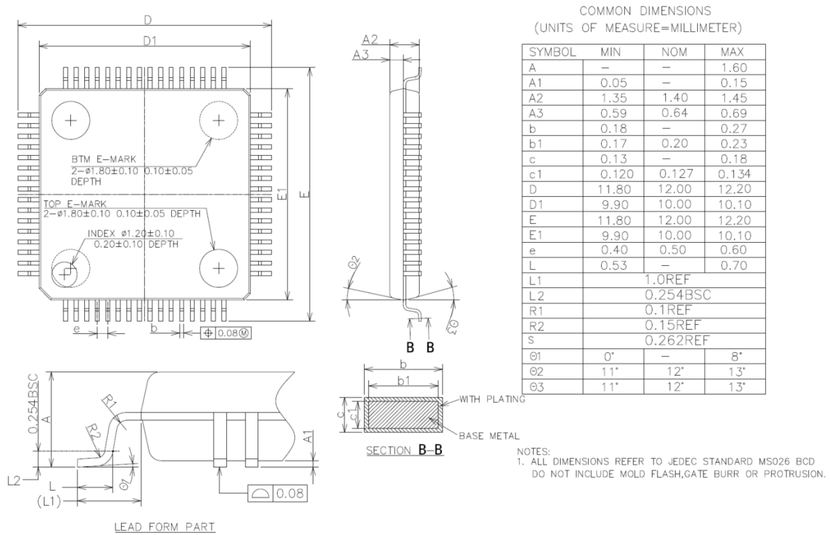
图 5-1: LQFP64 封装尺寸图
