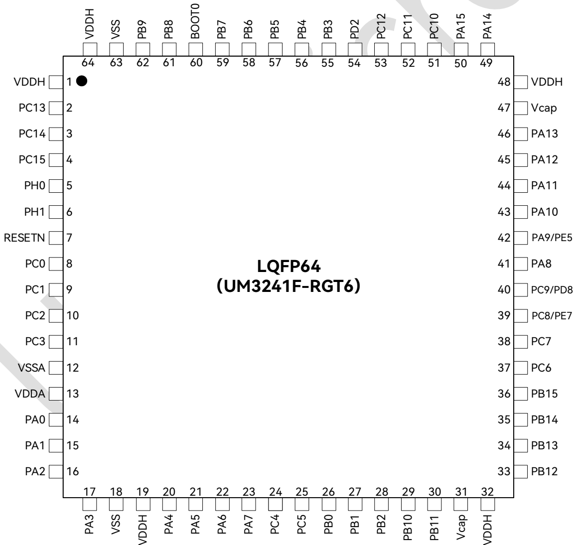
图 3-1: LQFP64 引脚分布图
