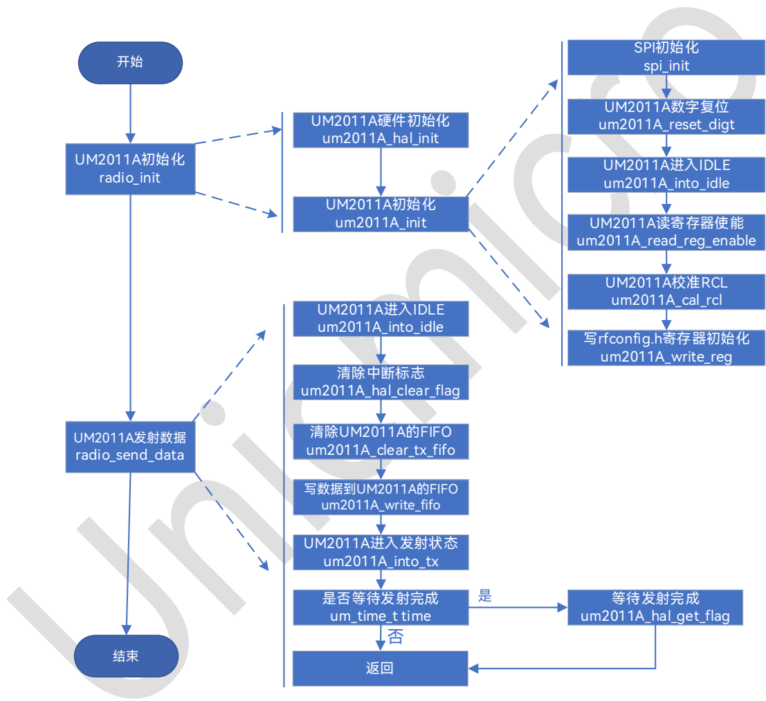
图 1-2: 发射数据流程图
