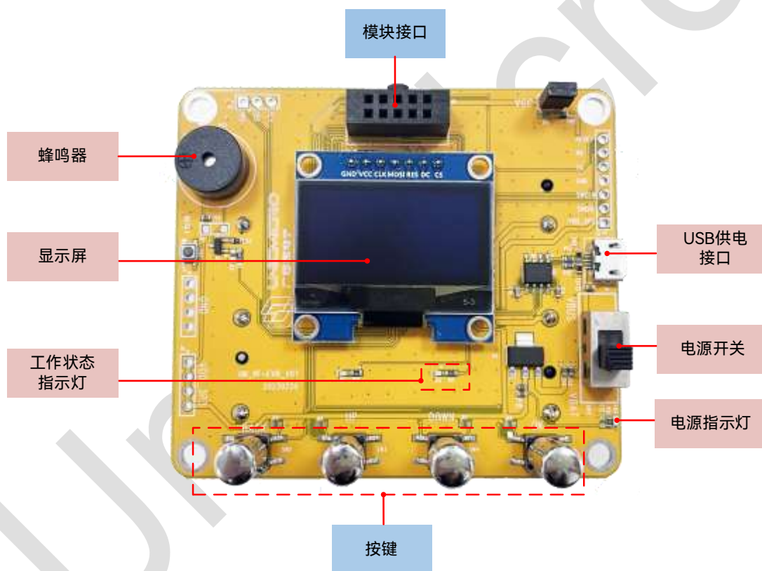
图 2-1：UM2006A RF-EVB 母板
