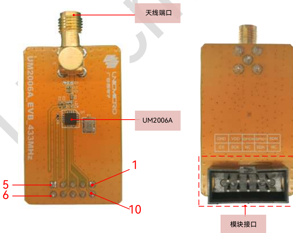
图 2-2：UM2006A RF-EVB 子板
