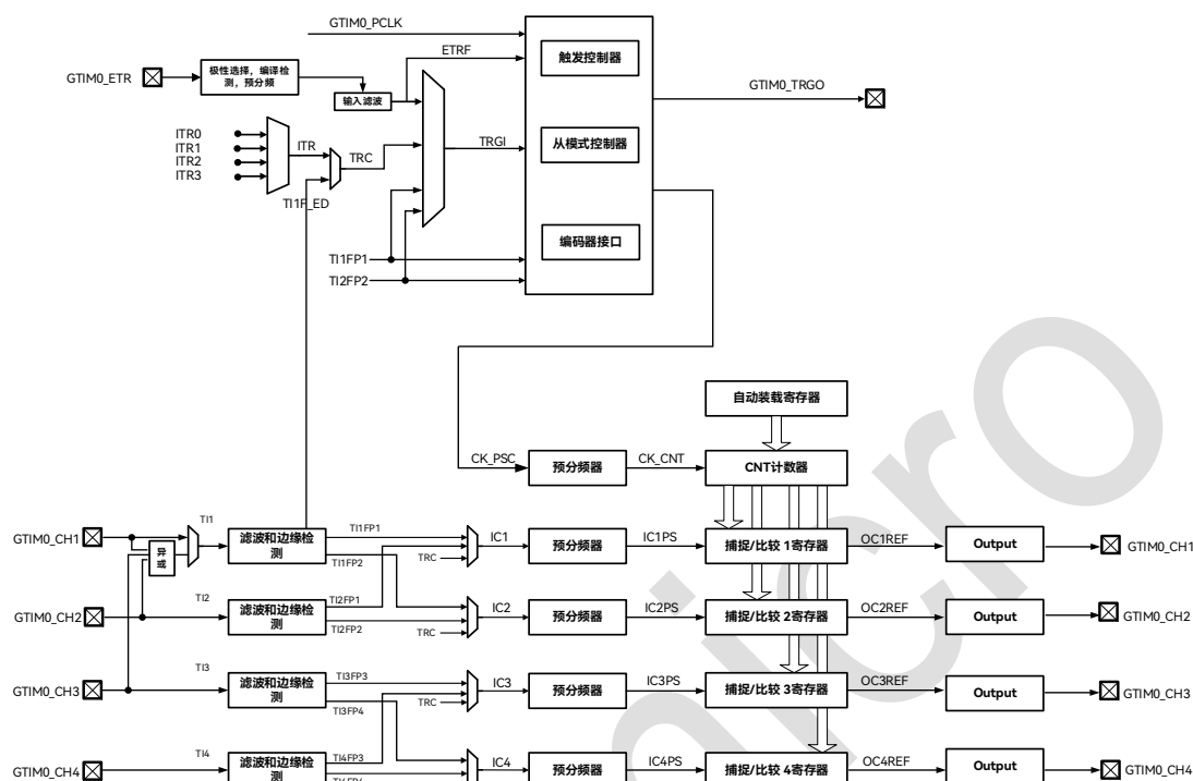
图 13-1: GTIMER 结构框图
