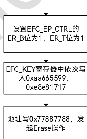
图 6-5: Chip 擦除操作流程
