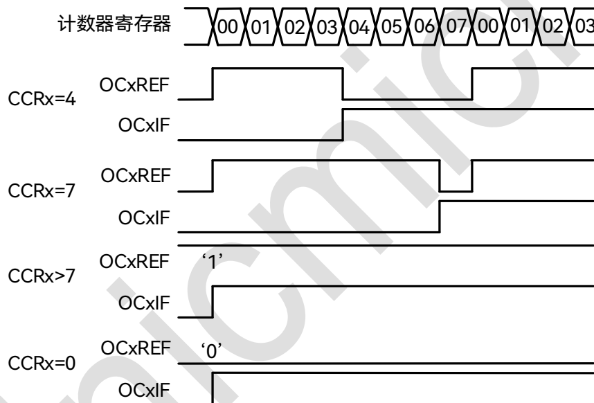
图 13-12: 边沿对齐的 PWM 波形 (ARR=7)
