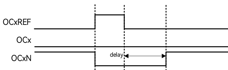
图 12-34: 死区波形延迟大于正脉冲
