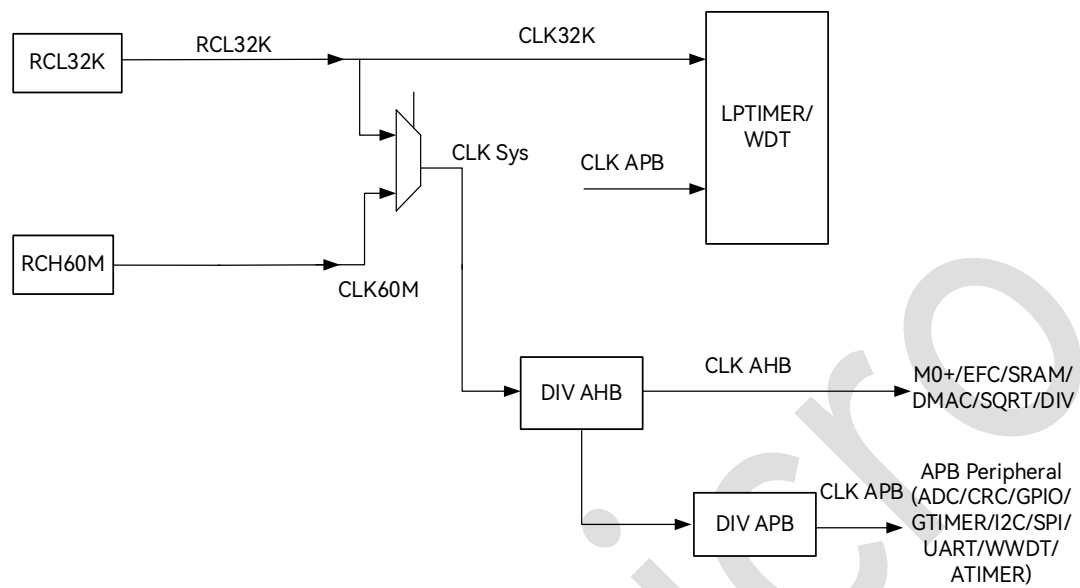
图 2-1：时钟架构图
