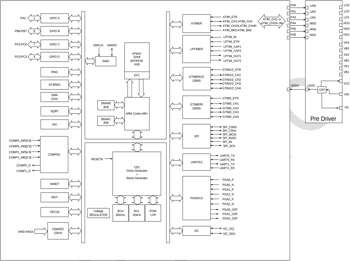
图 3-6: UM32MP56-H6U7 产品结构图
