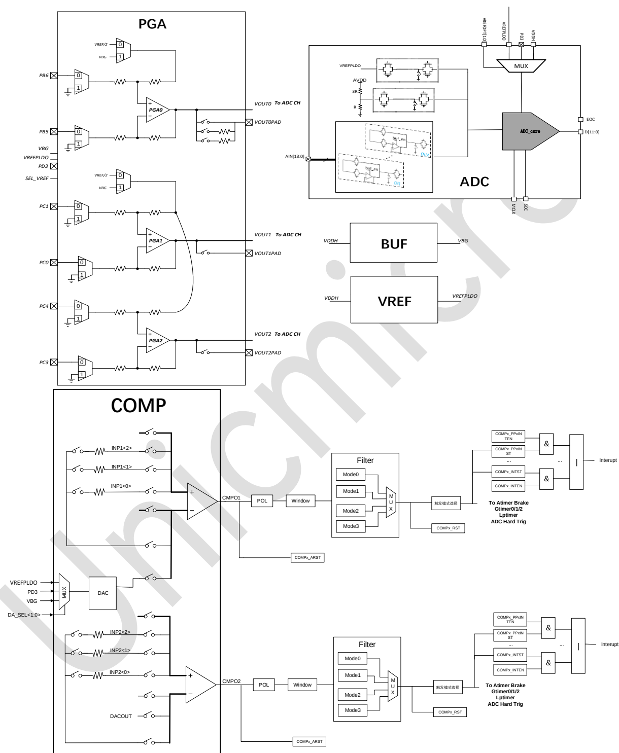
图 3-7：产品内部模拟信号连接
