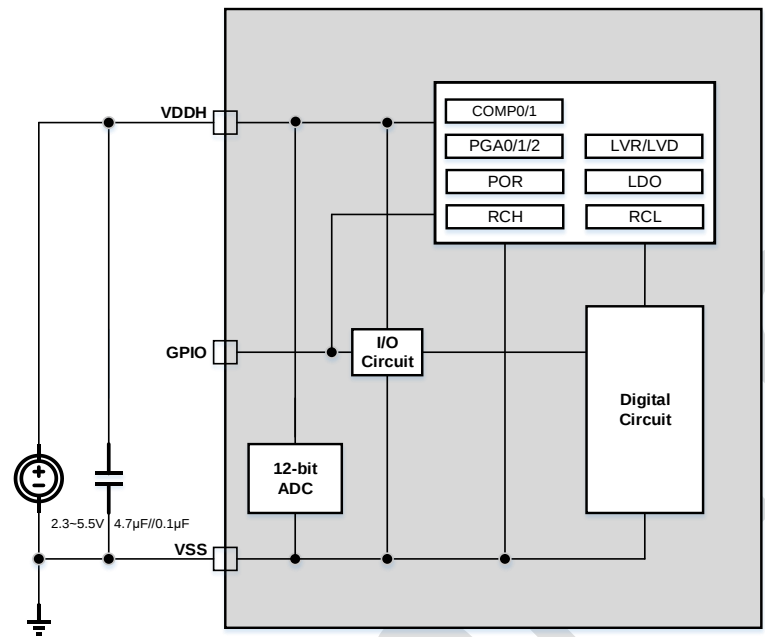
图 4-1：系统供电方案框图
