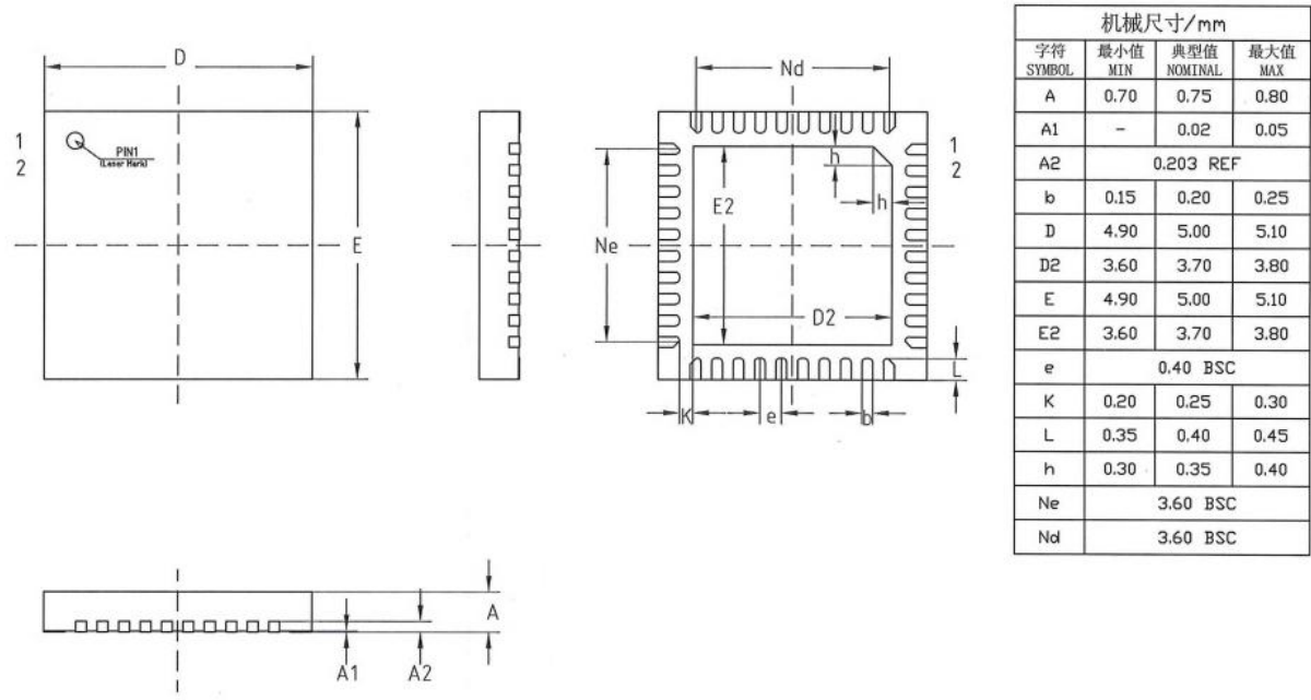
图 5-3: QFN40 封装尺寸图
