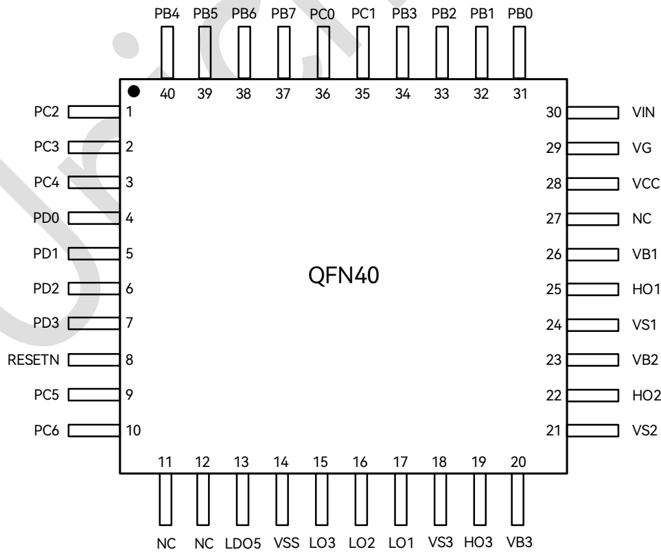
图 3-3: UM32MP56-H6U7 引脚分布图
