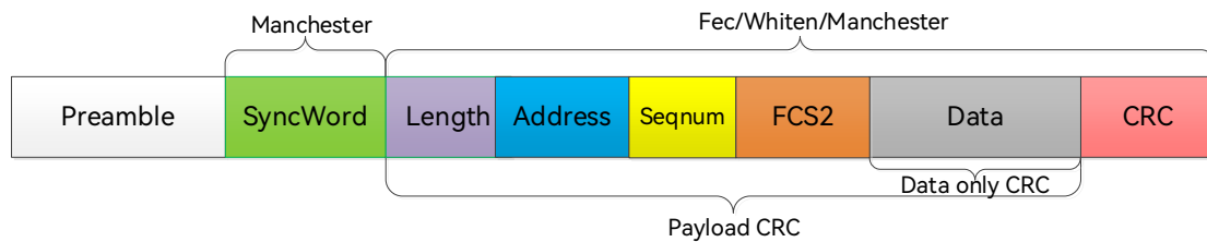
图 8-5: Mode 3 帧格式
