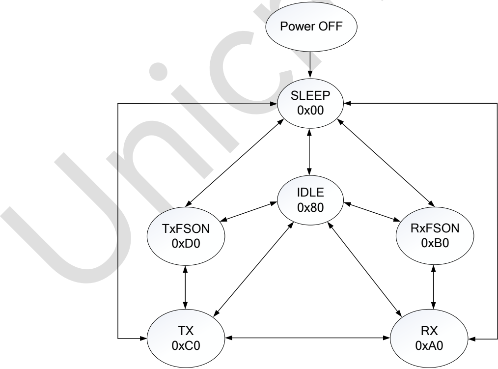
图 7-4：状态转换图
