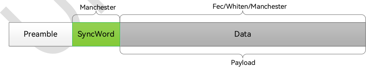
图 8-2：Mode 0 帧格式
