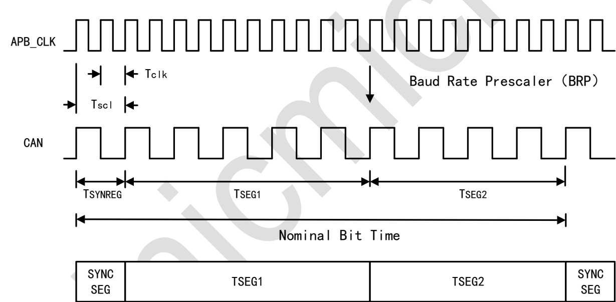
图 14-1：CAN 的位周期结构图
