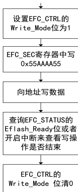
图 6-1：写操作流程
