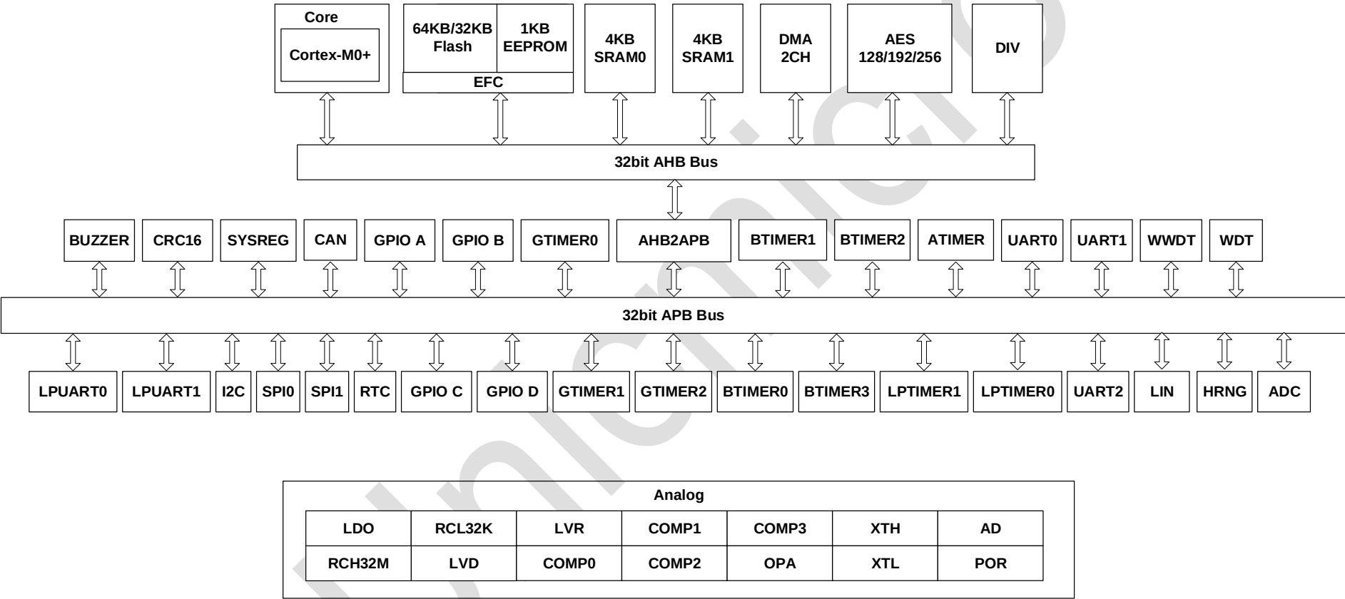
图 3-1：总线架构图
