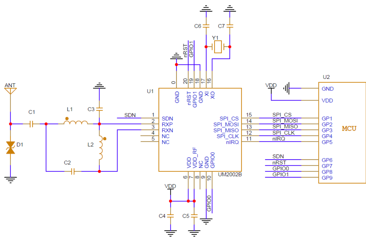
图 9-1：参考电路图
