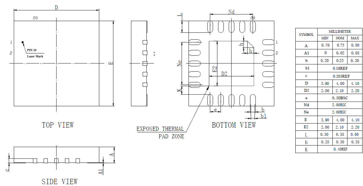
图 10-1：QFN20 封装图
