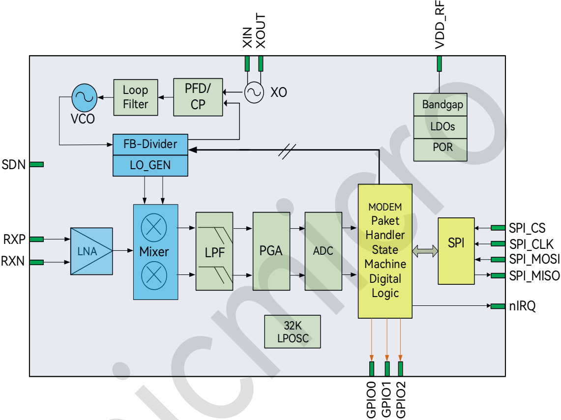
图 2-1：功能框图
