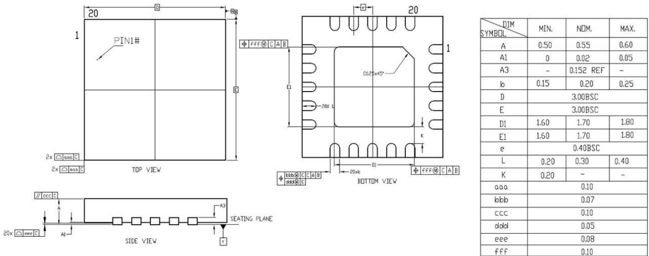
图 5-1: QFN20 封装图
