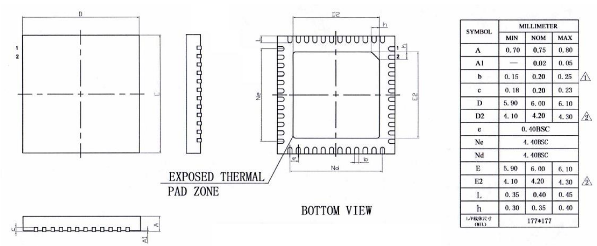
图 5-1: QFN48 封装尺寸图
