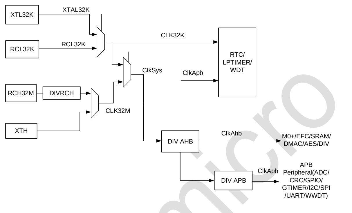
图 2-1：时钟架构图
