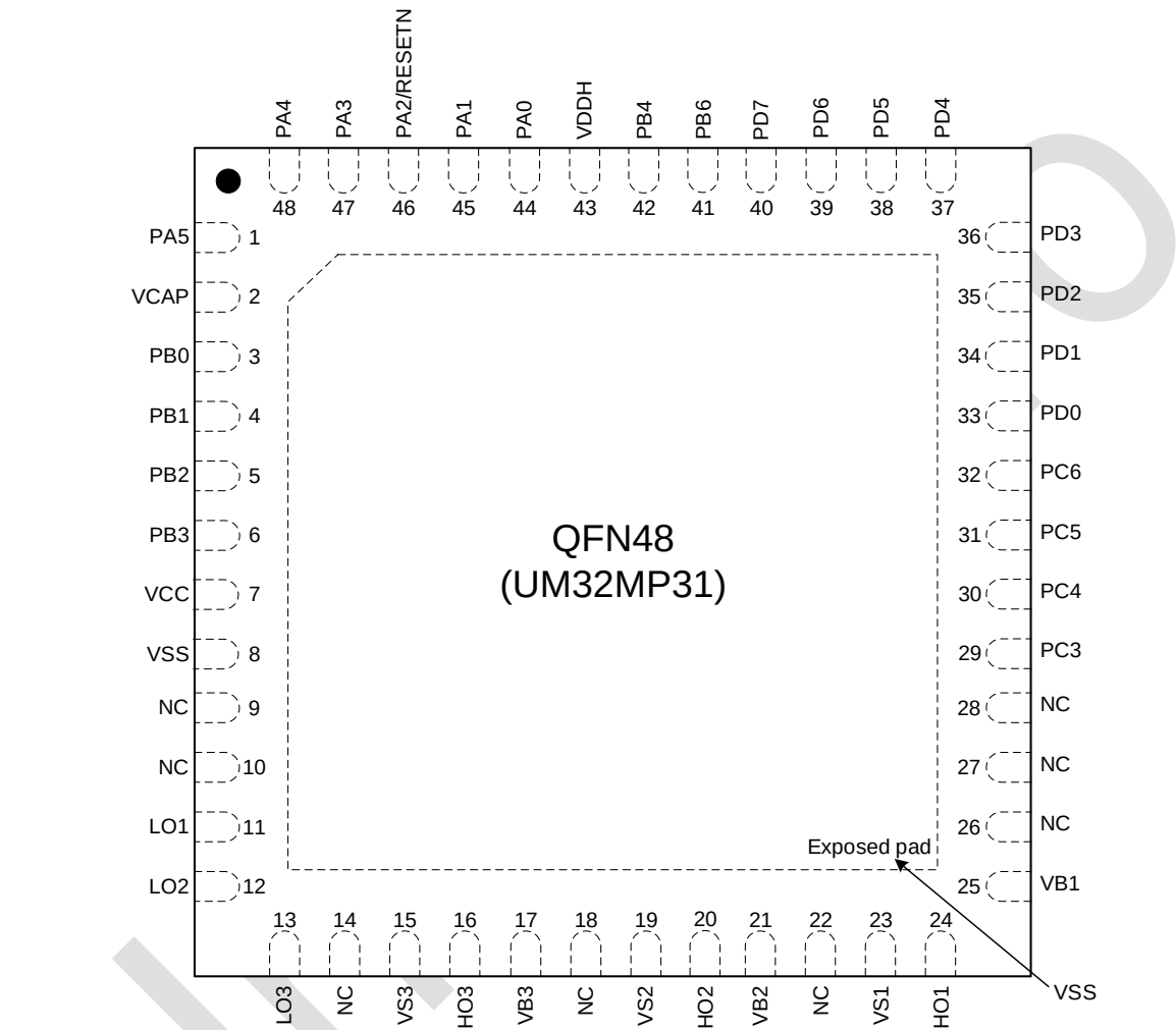
图 3-1：QFN48 引脚分布图
