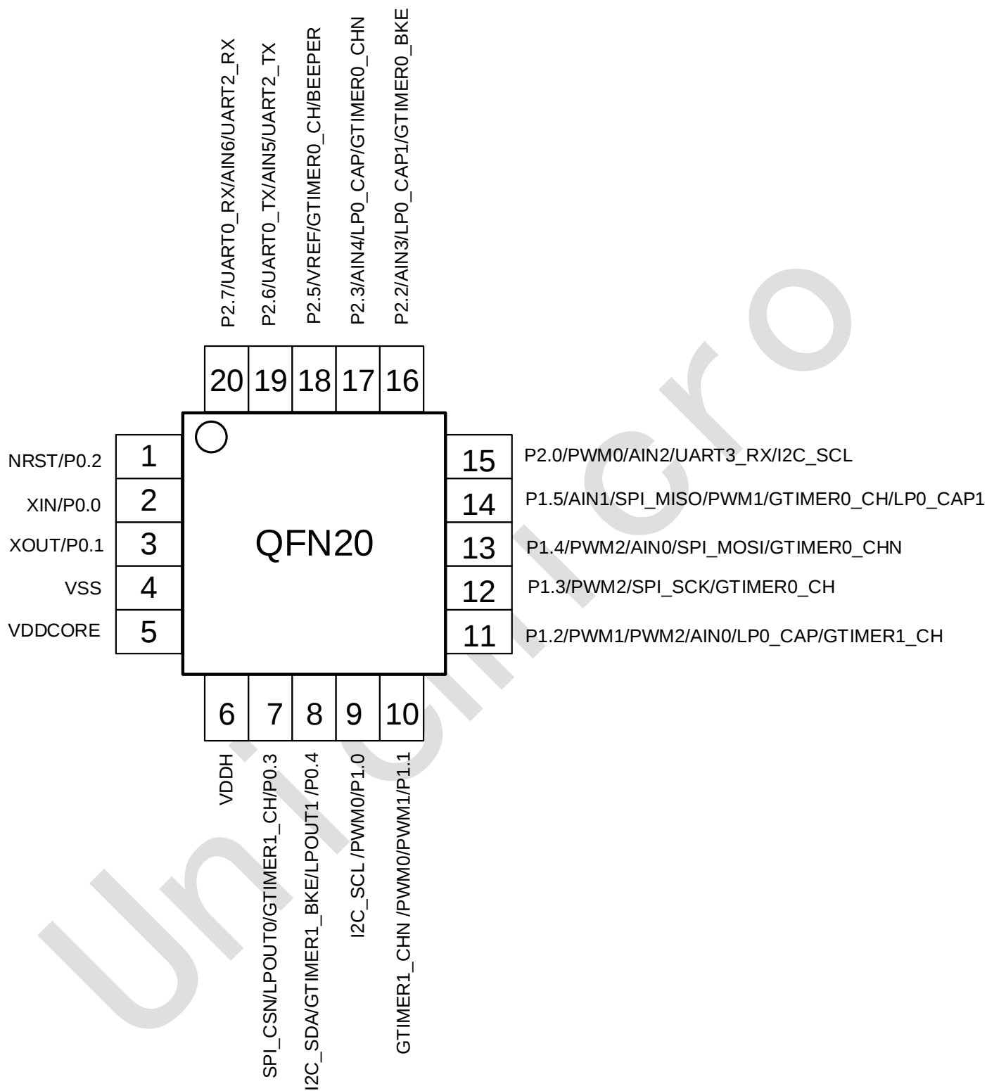
图 3-3: QFN20 封装管脚分布图
