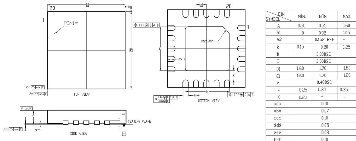
图 5-1: QFN20 封装图
