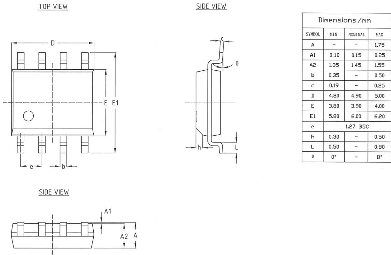
图 5-3: SOP8 封装图
