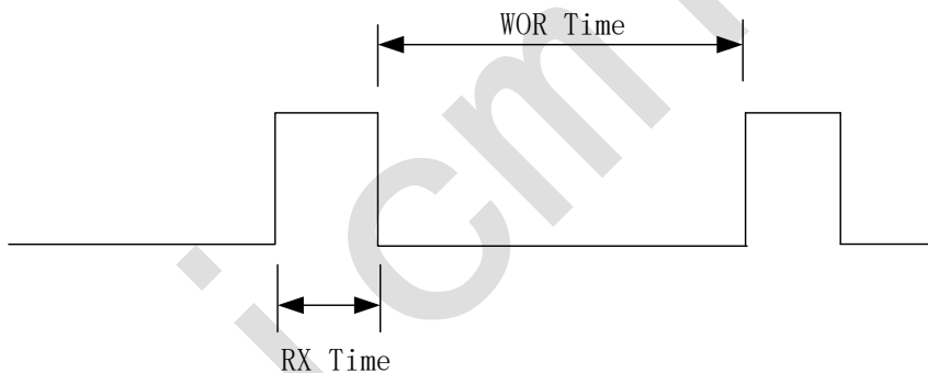
图 5-2：定时唤醒图
