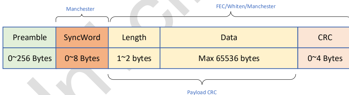
图 7-3: Mode 2 帧格式
