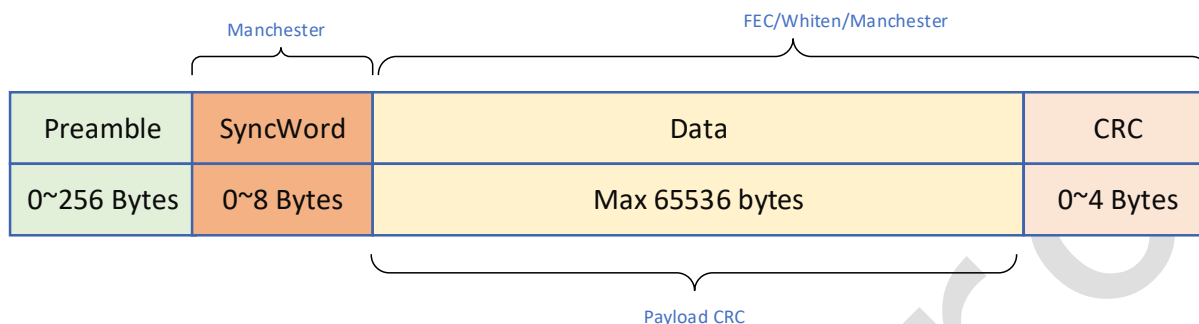
图 7-2: Mode 1 帧格式
