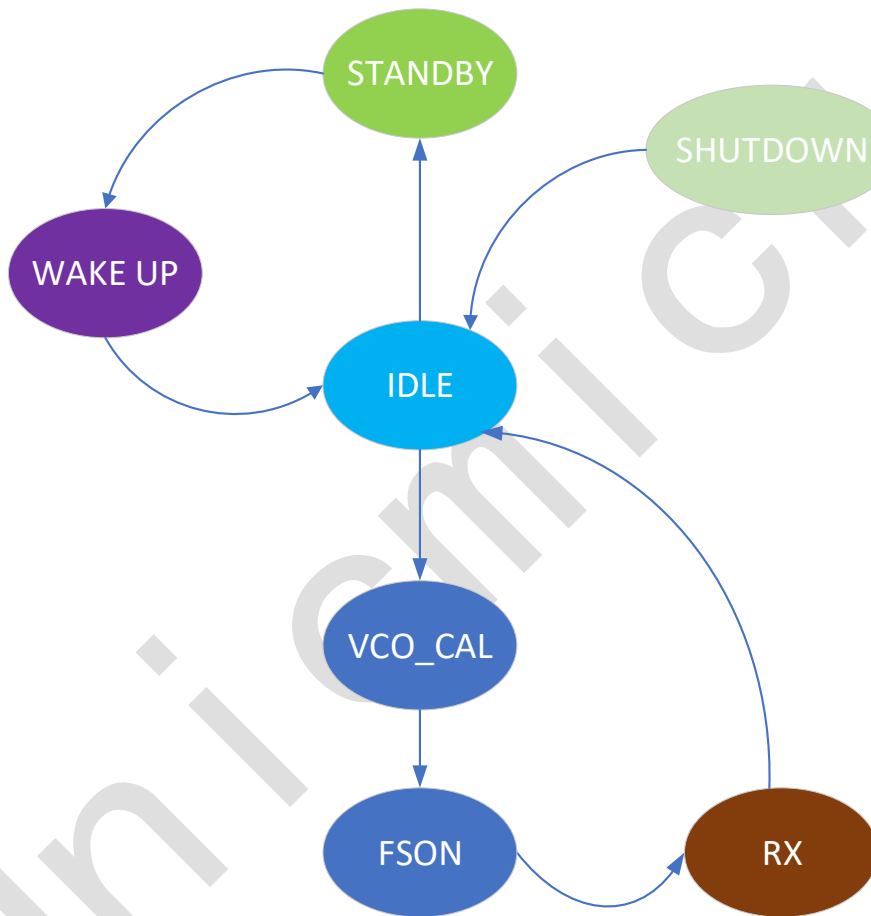
图 6-3：状态机控制图
