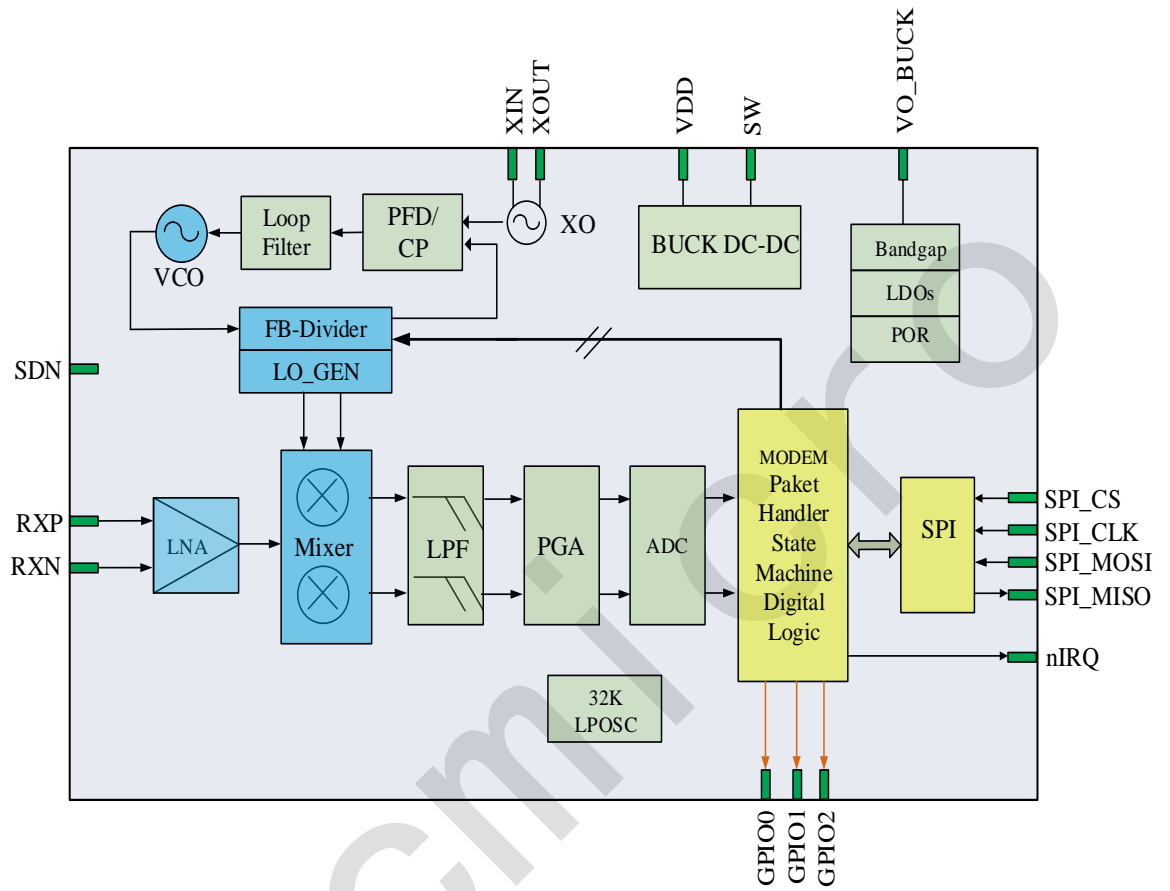
图 2-1: 功能框图
