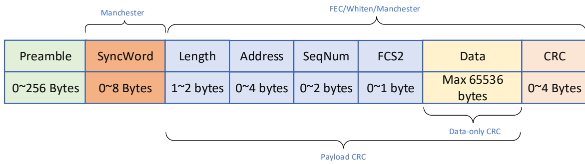
图 7-4: Mode 3 帧格式
