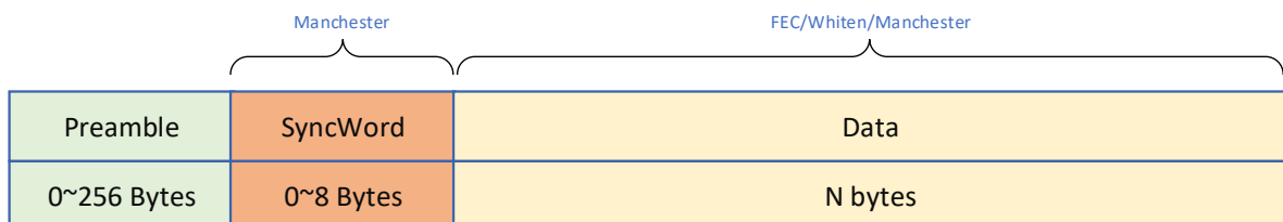
图 7-1：Mode 0 帧格式
