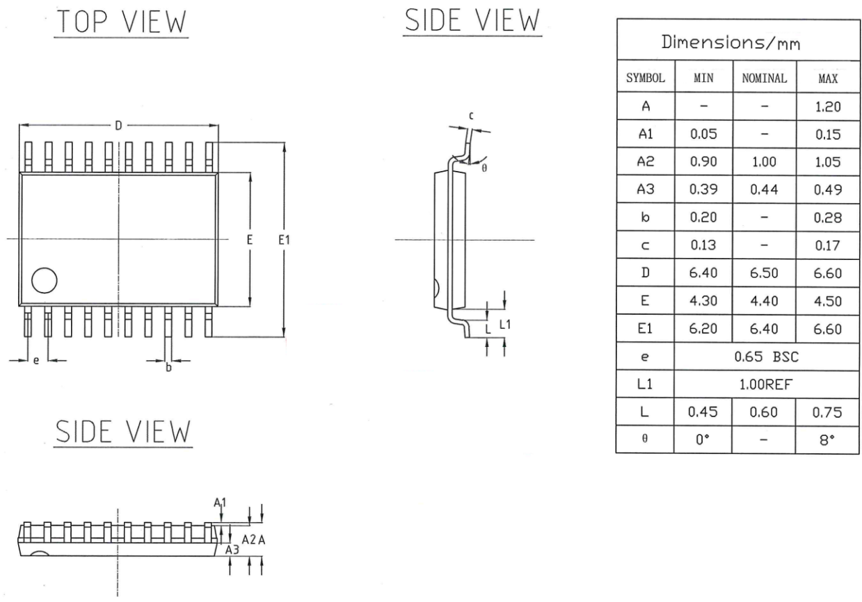
图 5-2：TSSOP20 封装图
