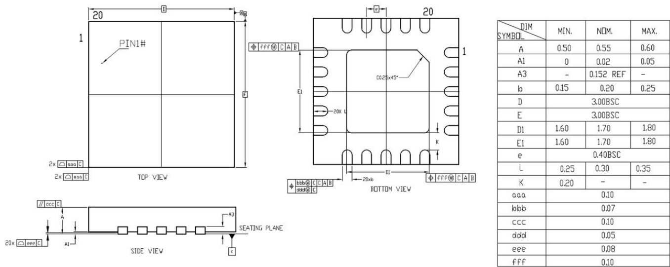
图 5-1: QFN20 封装图
