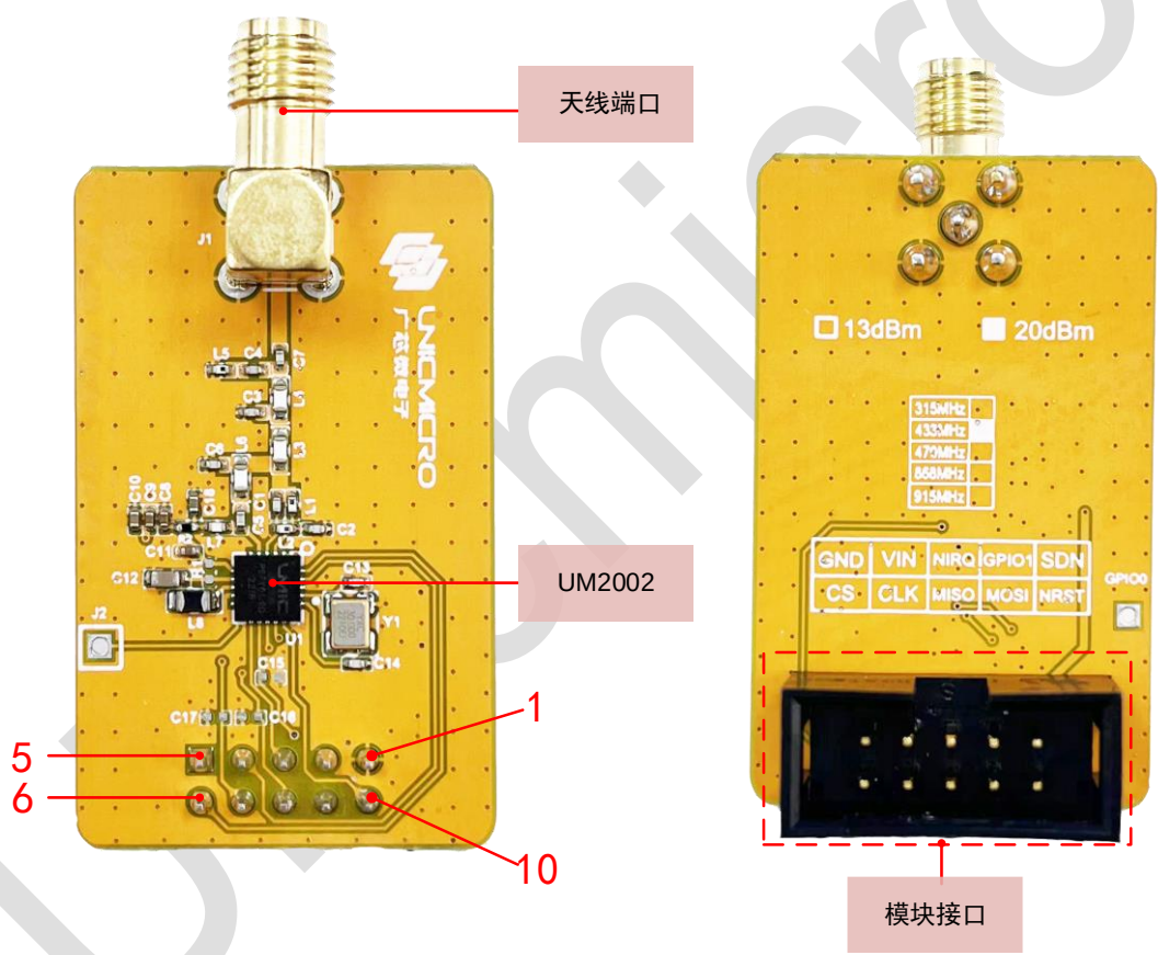
图 2-2: RF-EVB 子板
