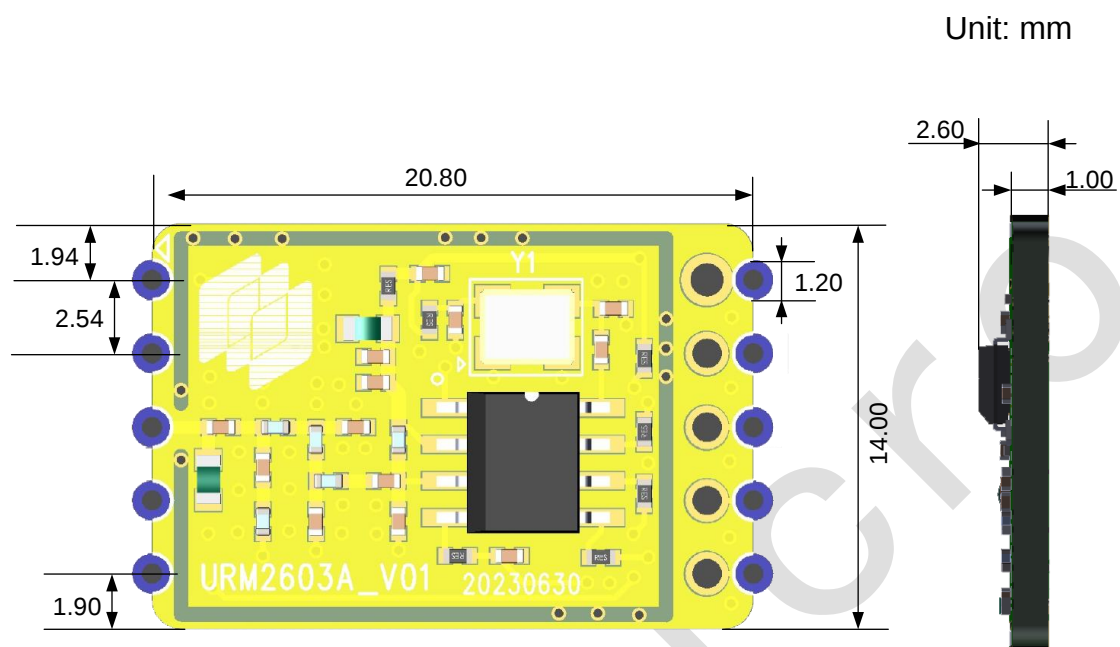
图 5-1: 模块尺寸图
