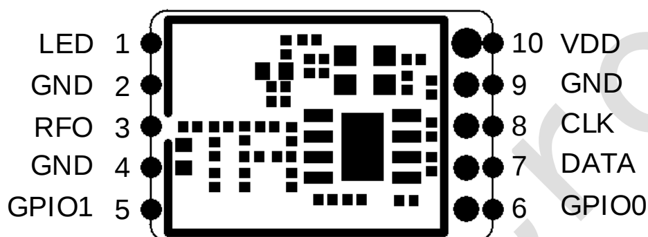
图 2-1: 引脚分布图
