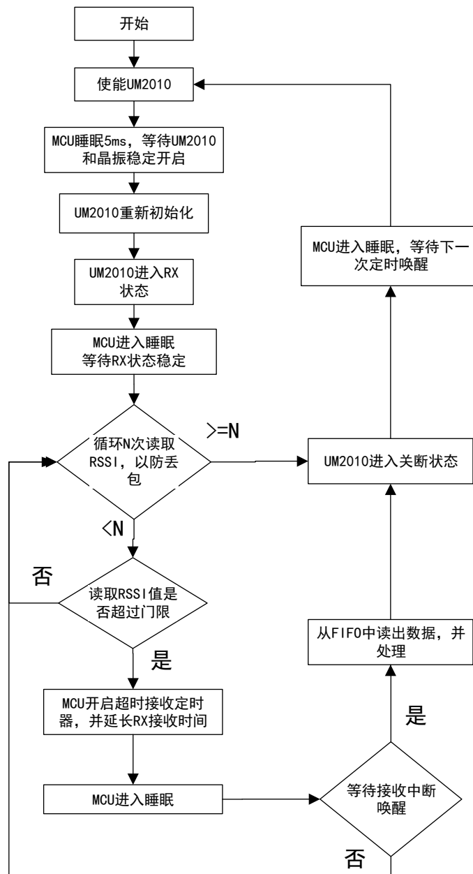
图 3-3: 接收检测 RSSI (Shutdown 模式) 流程图
