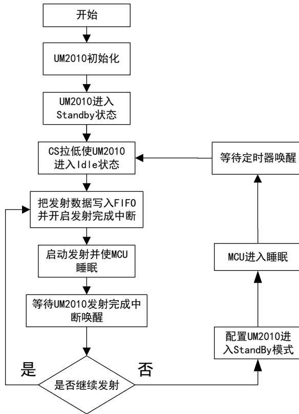
图 3-2: 低功耗发射 (StandBy 模式) 流程图
