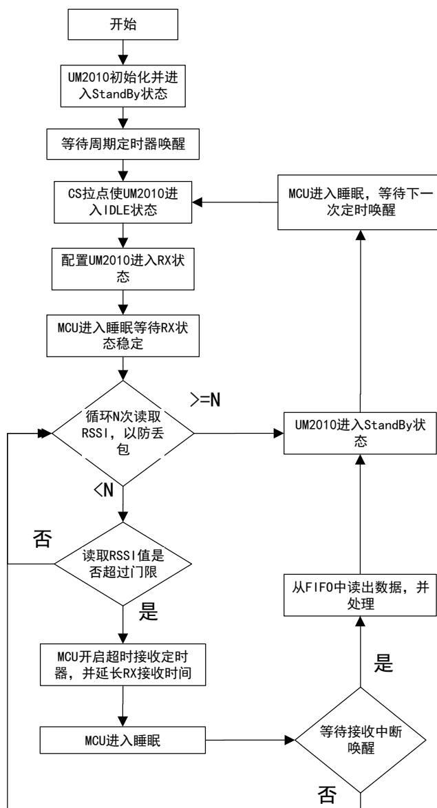
图 3-5: 接收检测 RSSI (StandBy 模式) 流程图
