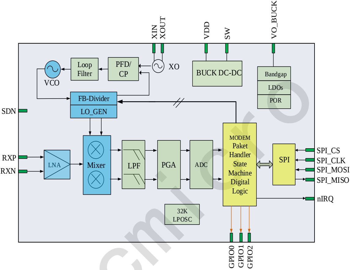
图 2-1：功能框图
