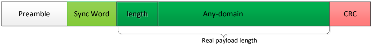
图 7-8：包模式 2
