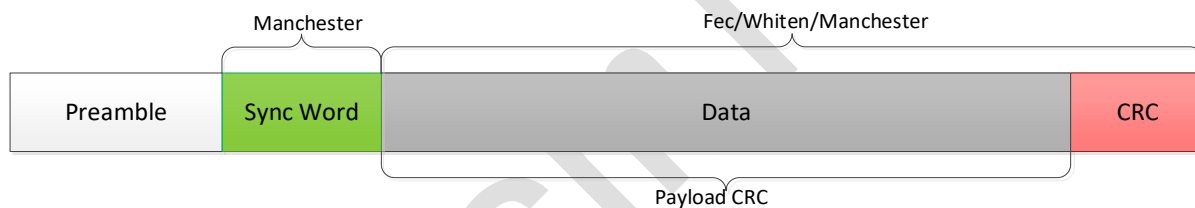
图 7-2: Mode1 帧格式
