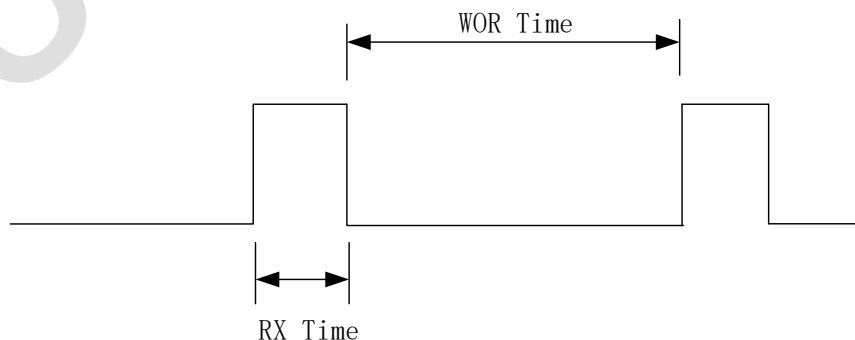
图 5-3：定时唤醒图
