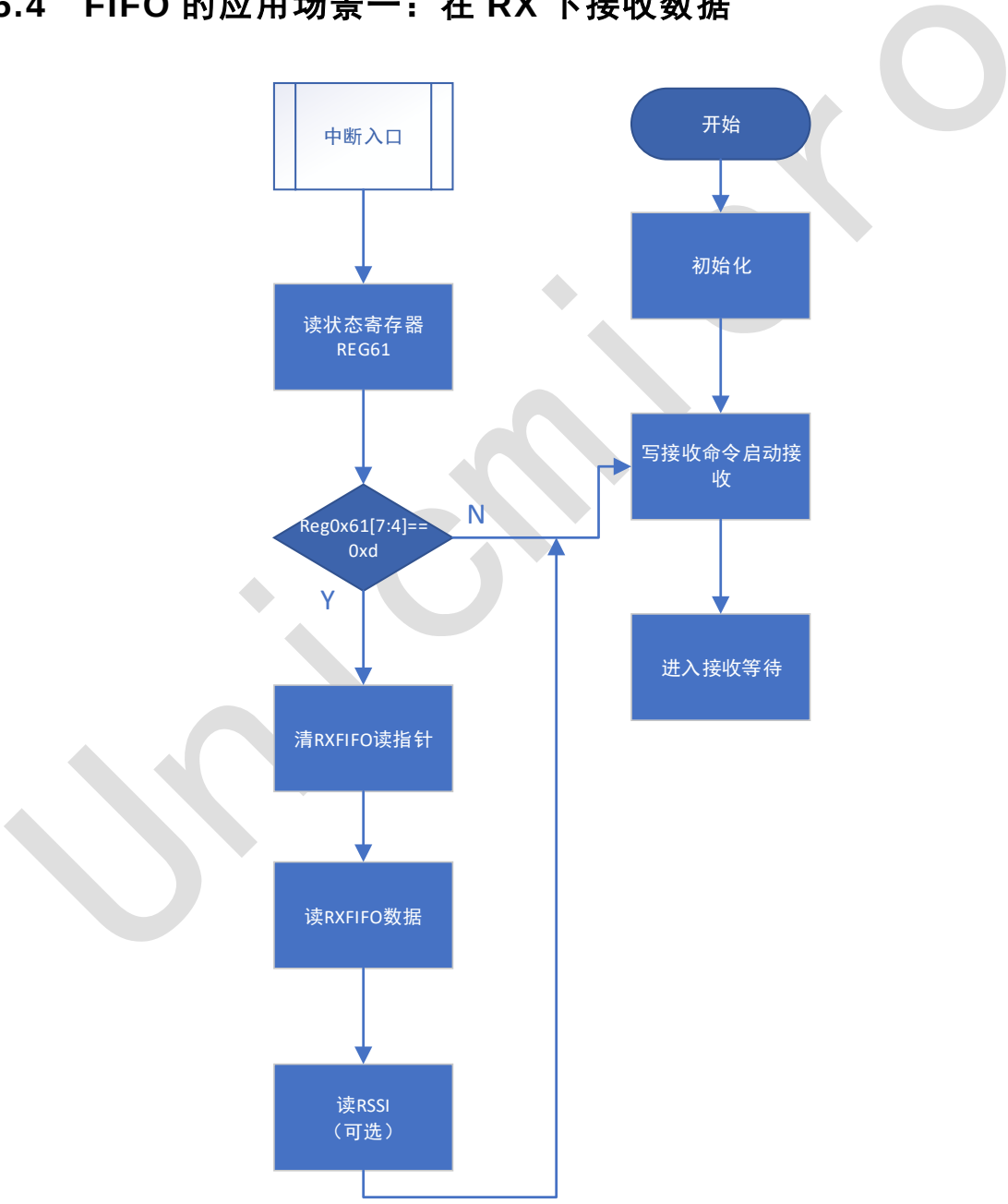
图 6-2：在 RX 下接收数据流程图
