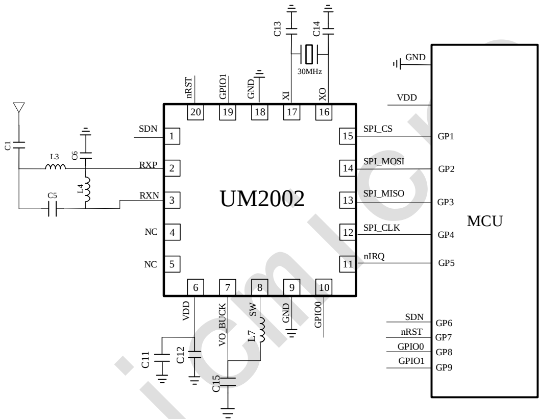
图 9-1：BUCK 模式应用参考电路图
