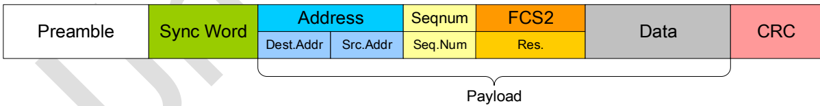
图 7-10：固定长度包格式
