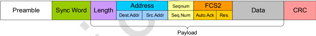
图 7-13: 可变长度包格式, Address 存在, Address 在 Length Byte 之后
