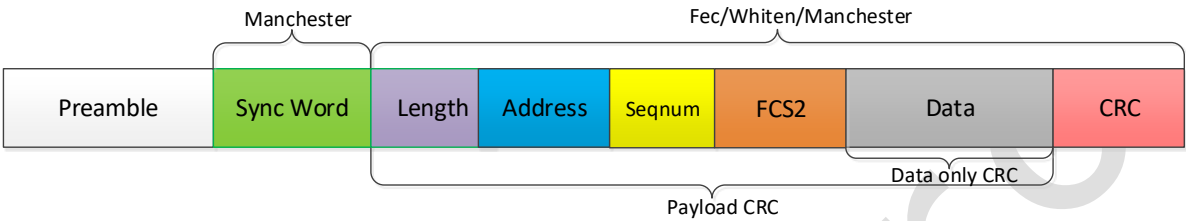
图 7-4：Mode3 帧格式
