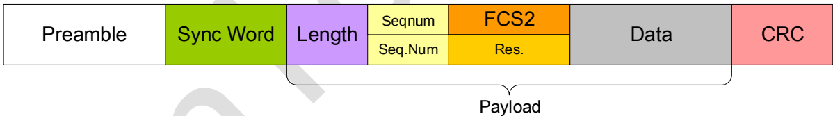
图 7-11：可变长度包格式，Address 不存在
