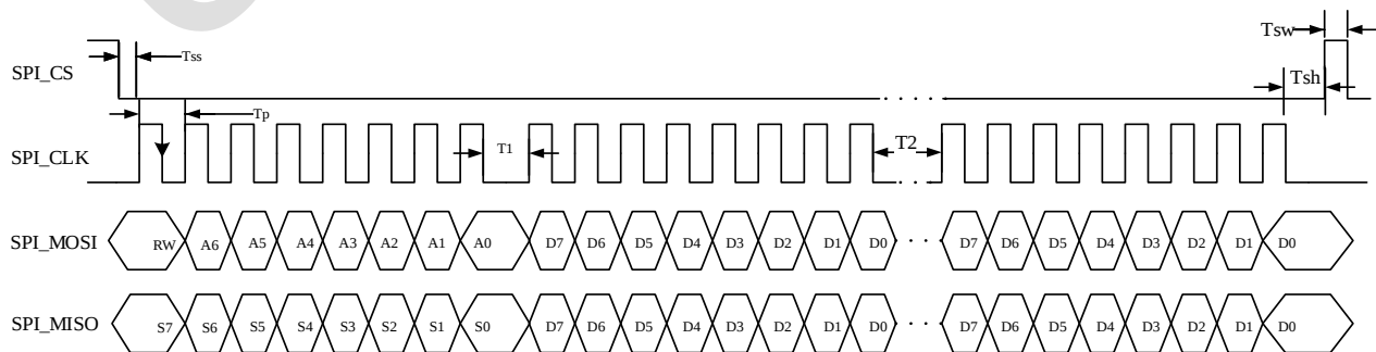
图 8-2: SPI 读写 FIFO 时序图
