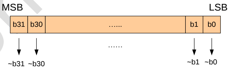
图 7-15: CRC_INV
