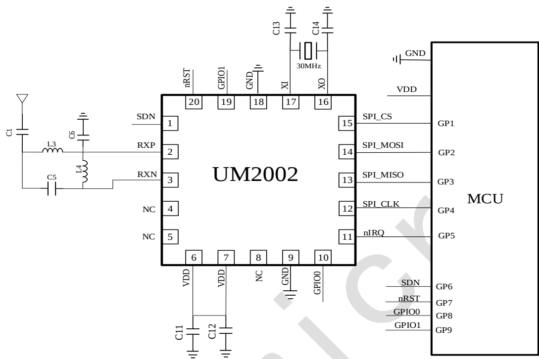
图 9-2：非 BUCK 模式应用参考电路图
