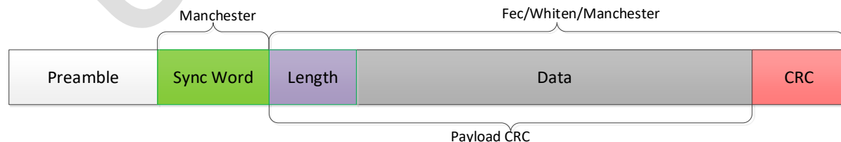
图 7-3: Mode2 帧格式
