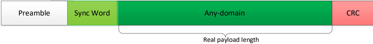
图 7-7: 包模式 1
