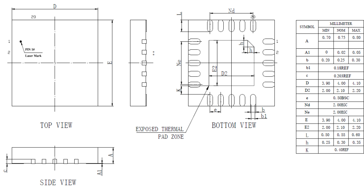
图 11-1：QFN20 封装图
