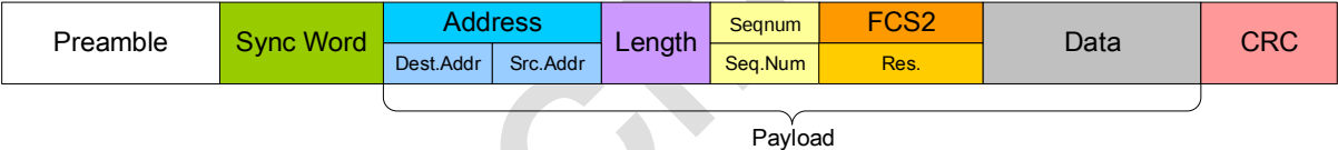
图 7-12：可变长度包格式，Address 存在，Address 在 Length Byte 之前
