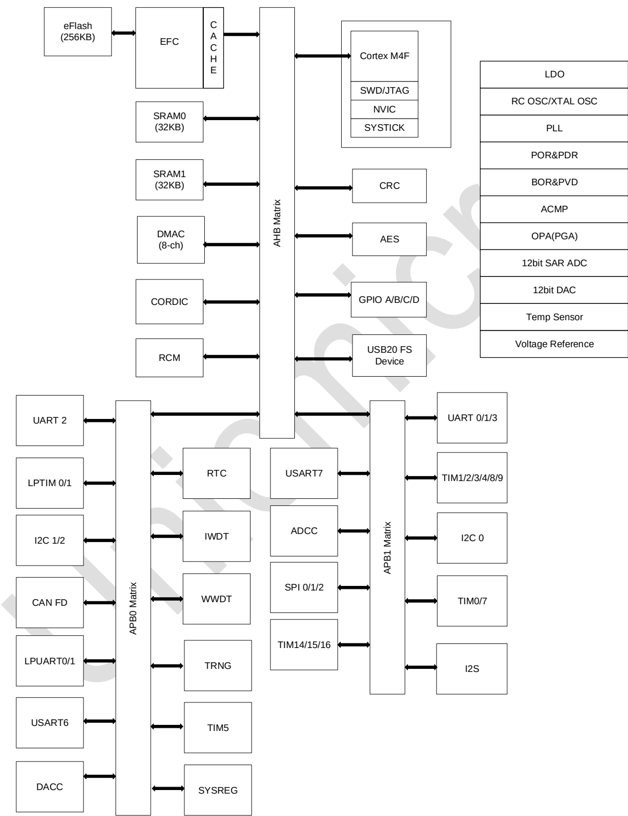
图 1-1：功能框图
