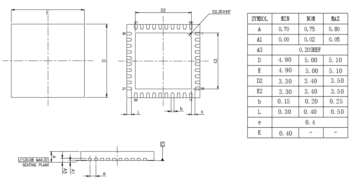
图 5-5：QFN40 封装尺寸图
