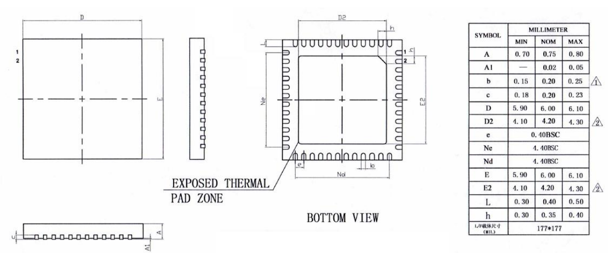
图 5-4：QFN48 封装尺寸图
