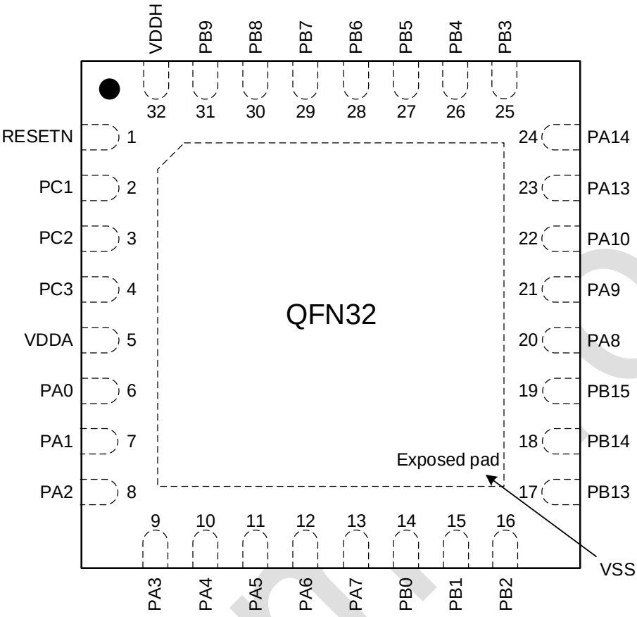
图 3-6: QFN32 引脚分布图
