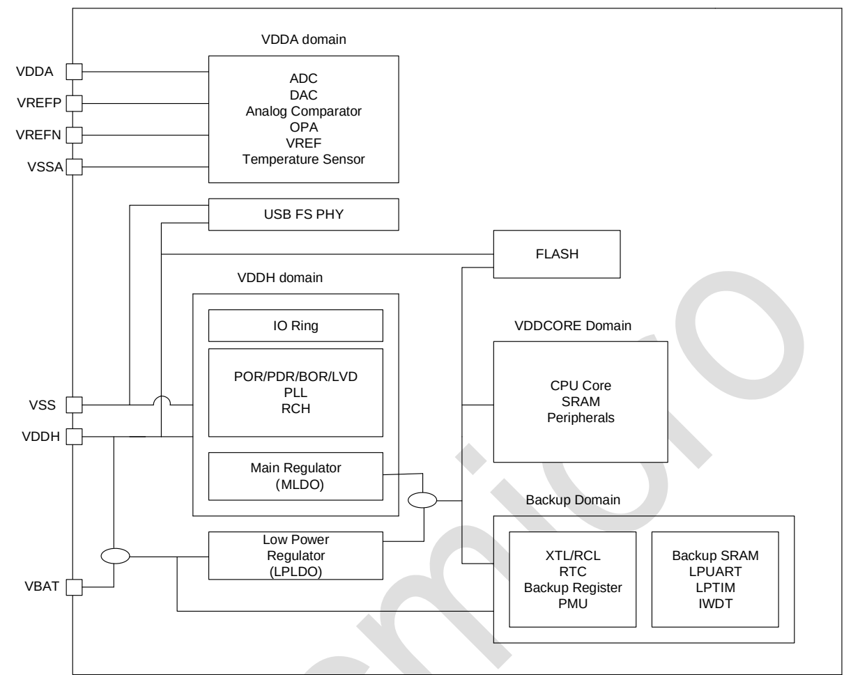
图 4-1：系统供电方案框图
