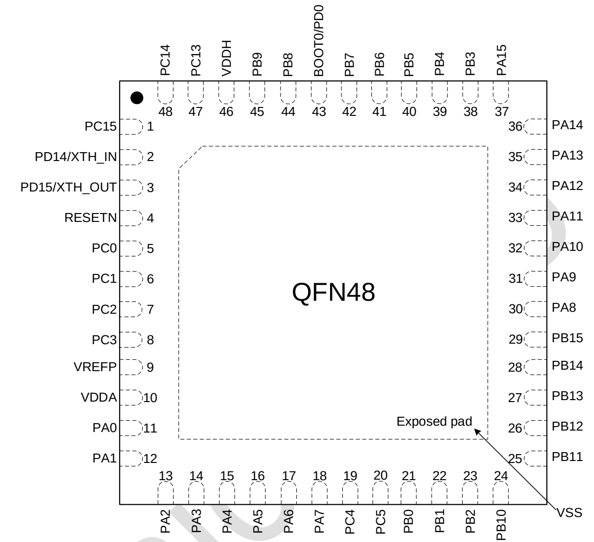
图 3-4: QFN48 引脚分布图
