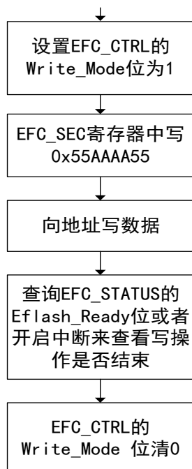
图 6-1: 写操作流程
