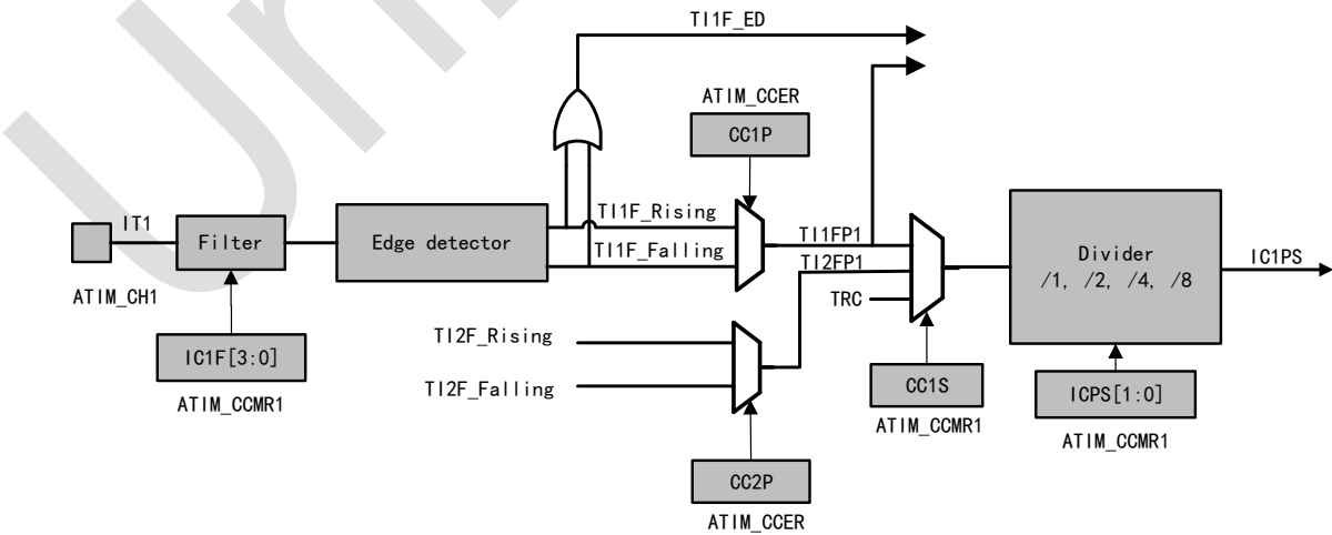
图 16-2：捕获/比较通道(通道 1 输入部分)
