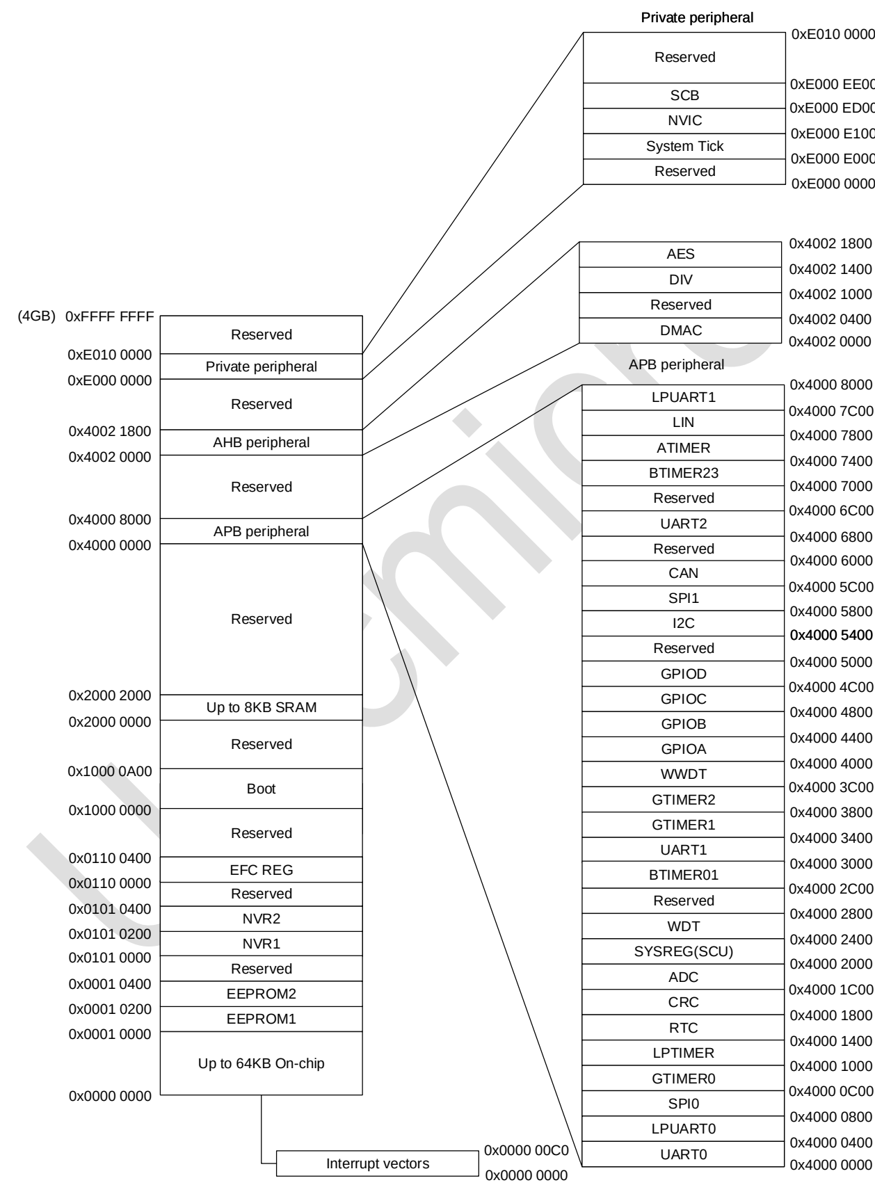
图 3-2：存储器地址映射图
