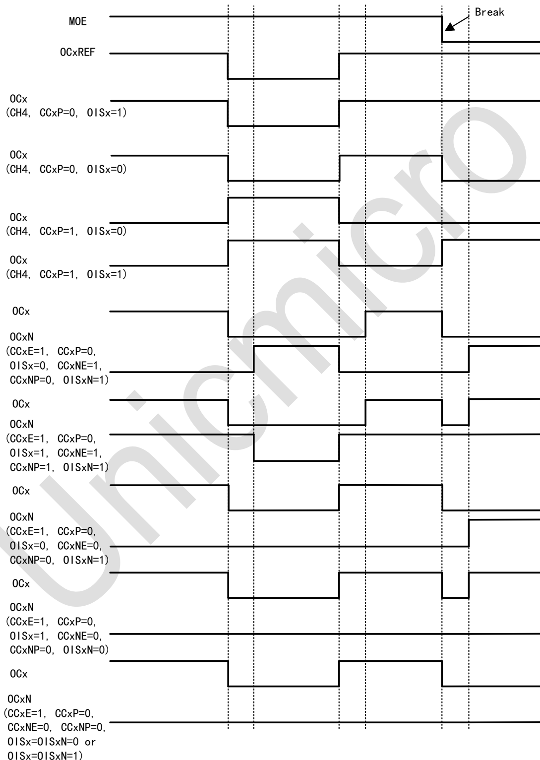
图 16-10：响应刹车的输出
